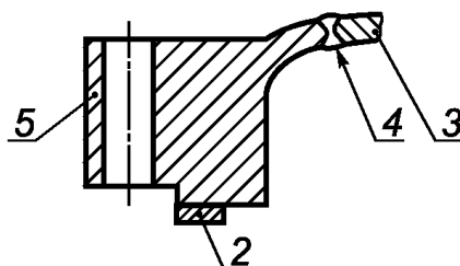
b - конструкция фланец-днище
