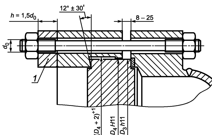
Рисунок 6 - Размеры и отклонения размеров деталей плавающей головки
