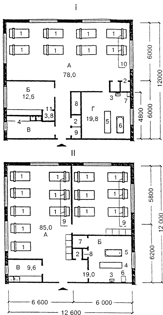
I - планировочная схема жилых комнат жилой ячейки типа 1в для лежащих детей с сохранным интеллектом
