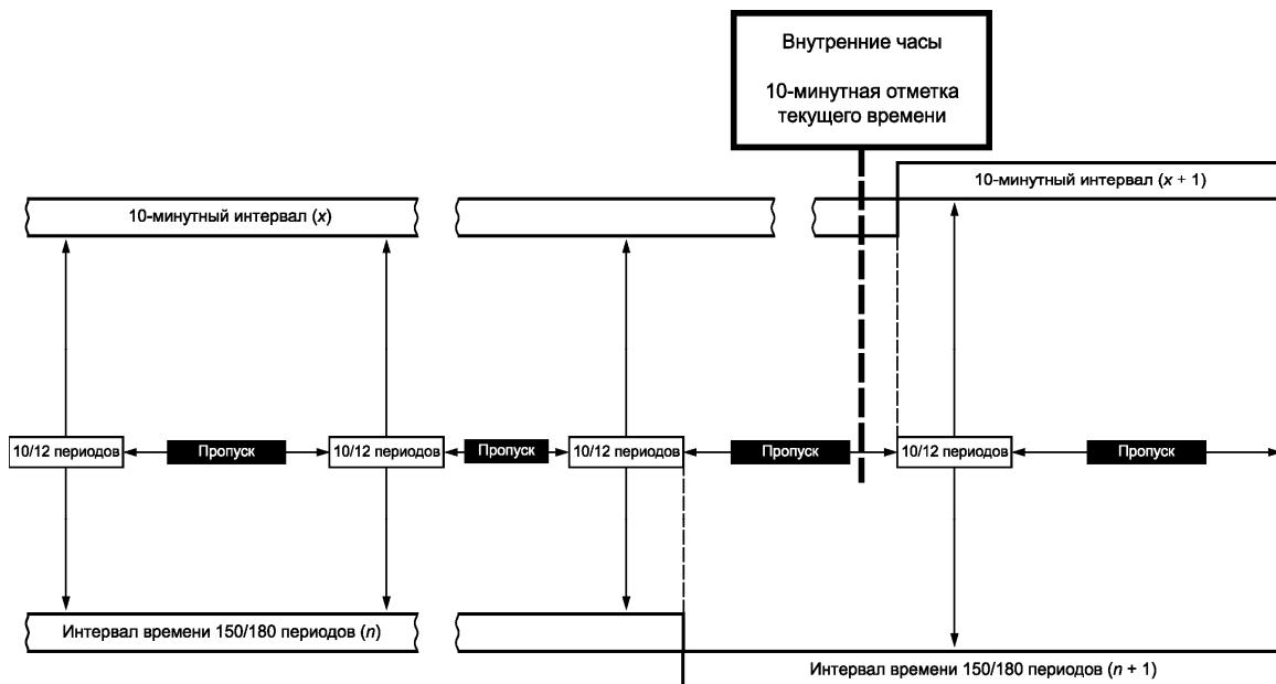
Рисунок 4. Синхронизация объединенных интервалов для класса S: измерение показателей КЭ, для которых пропуски допускаются
