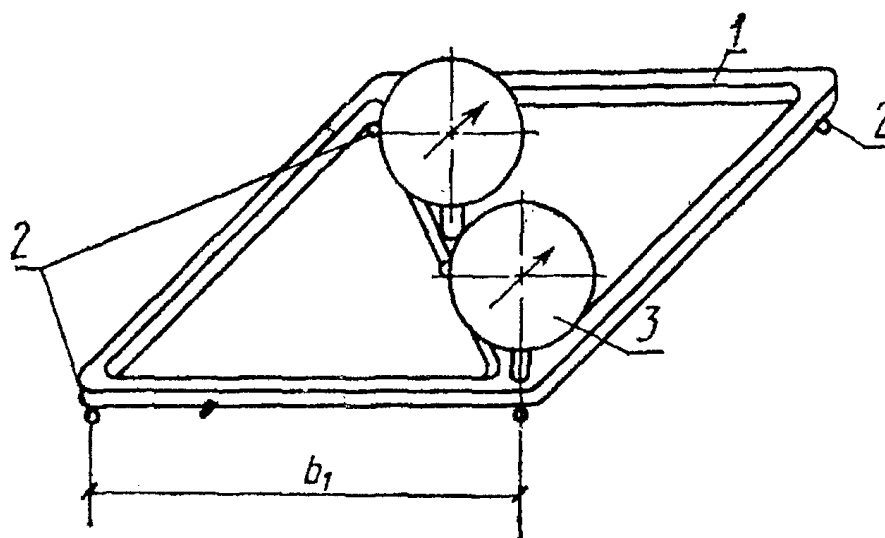
Схема прибора для измерения отклонений от плоскостности
