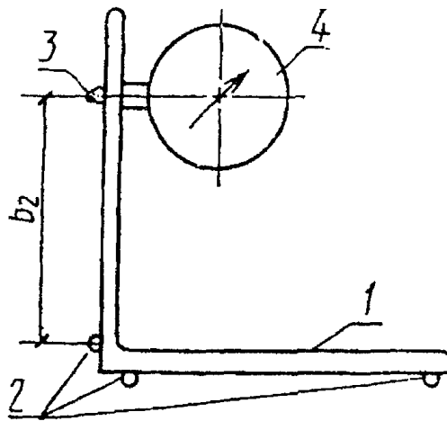
1 - корпус (угольник); 2 - опора; 3 - измерительный стержень индикатора; 4 - индикатор; b_2 - база прибора
