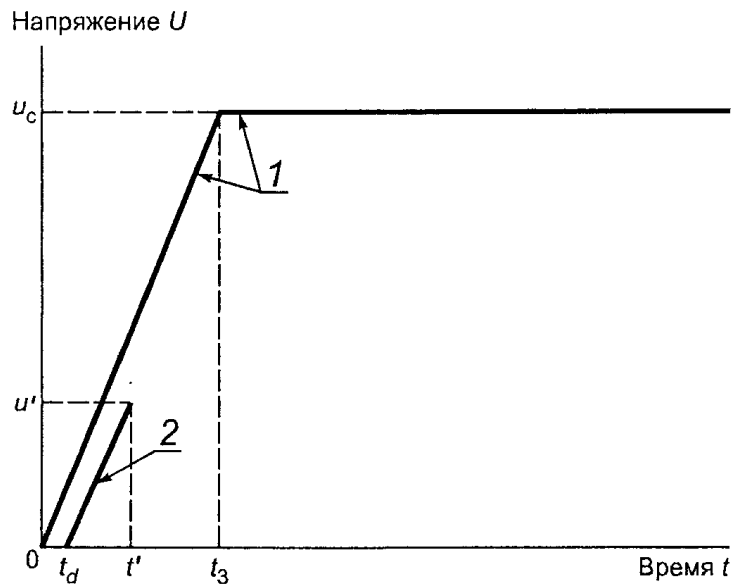
1 - условная граничная линия ПВН; 2 - линия запаздывания ПВН (параллельная граничной линии)
