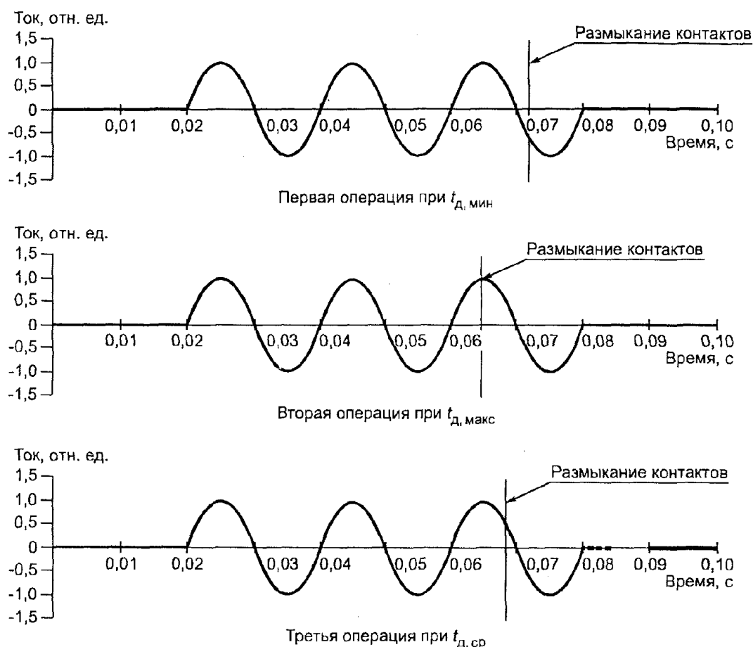
Рисунок 11. Регулирование момента размыкания контактов относительно фазы тока при однополюсном отключении
