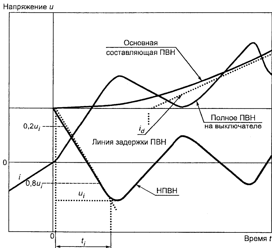
Рисунок 6. Начальная часть переходного восстанавливающегося напряжения (НПВН)
