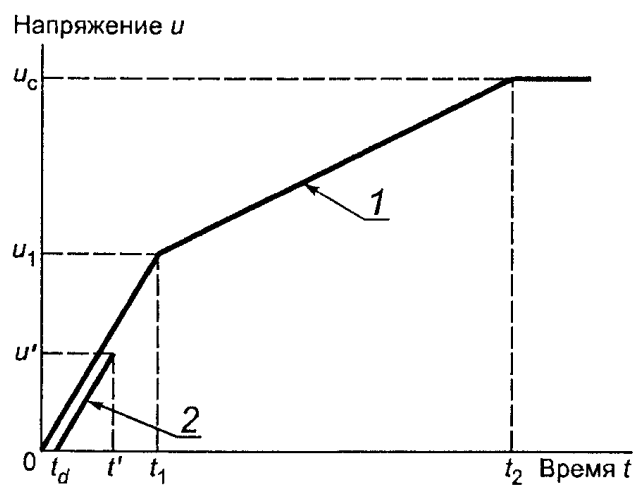
1 - условная граничная линия ПВН; 2 - линия запаздывания ПВН (параллельная граничной линии)
