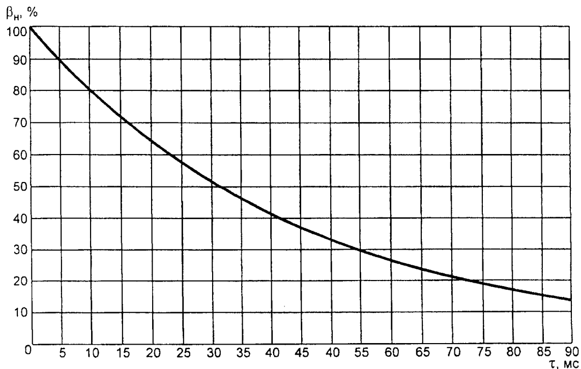
Рисунок 3. Содержание апериодической составляющей в процентах
