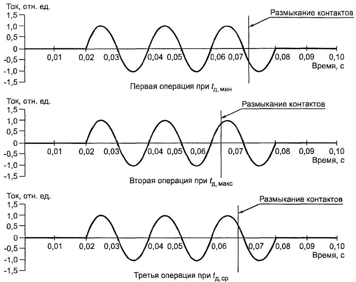
Рисунок 13. Регулирование момента размыкания контактов относительно фазы тока при однополюсном отключении симметричного тока в режимах Т10, Т30, Т60, Т100с, Тсr1, Тсr2, Тсr3, ОР2, L90, L75, L60 выключателями U_{ном} \geq 110 кВ
