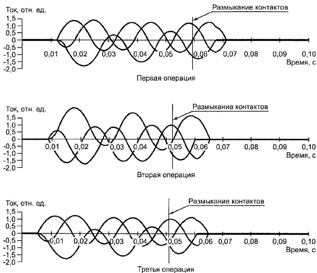
Рисунок 10. Регулирование моментов инициирования тока и размыкания контактов относительно фазы тока при трехполюсном отключении тока в режиме T100a
