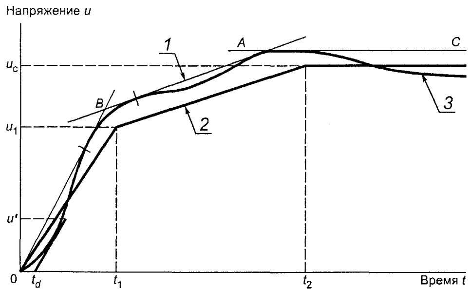
Рисунок 7. Построение огибающей ПВН, определяемого двумя параметрами
