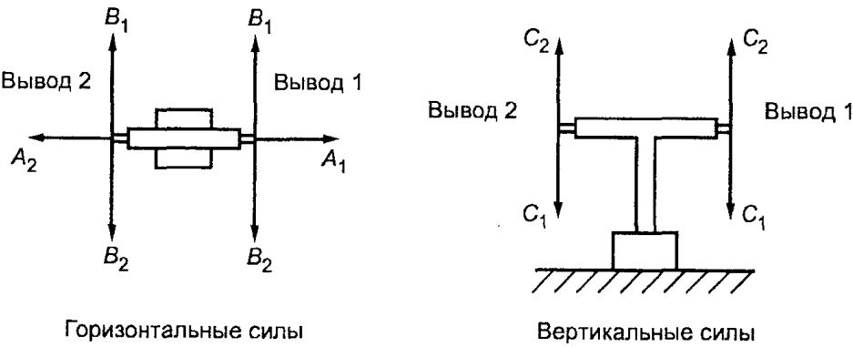
а) Статические нагрузки на выключатель
