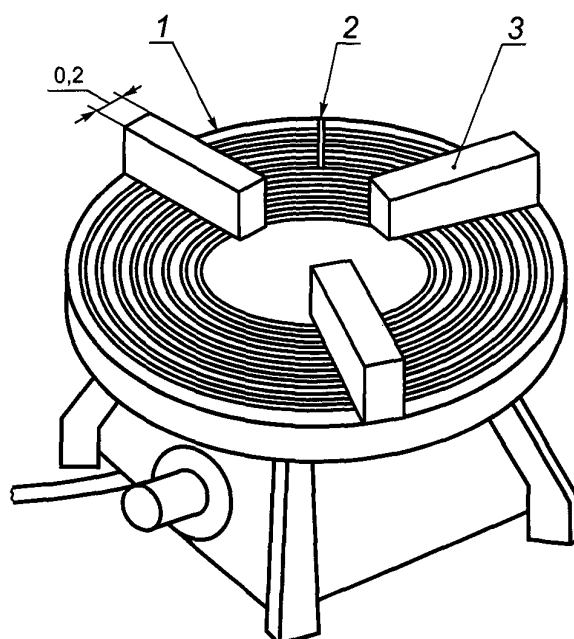
1 - плита; 2 - термопара; 3 - деревянные бруски
