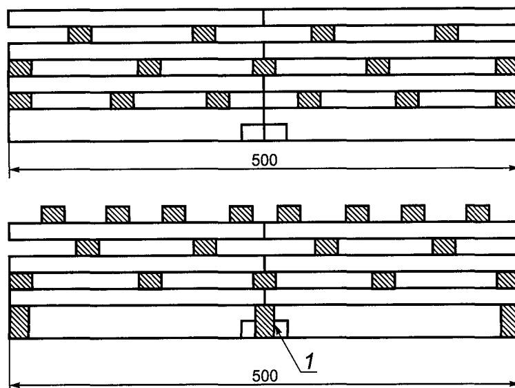
1 - контейнер для легко воспламеняющейся жидкости
