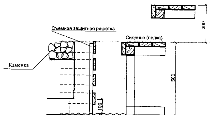
Рис. 6.3. Планировочные схемы саун, доступных для инвалидов
