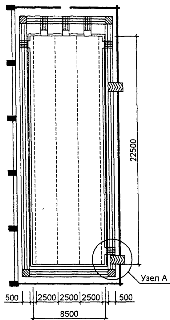
Ванна для терапевтических занятий
