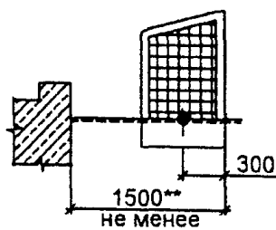
Свободно плавающие ворота
