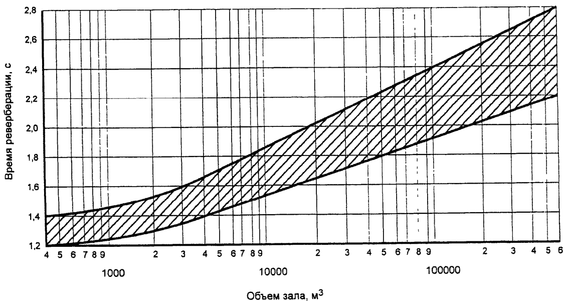
Рисунок 9.1. График времени реверберации
