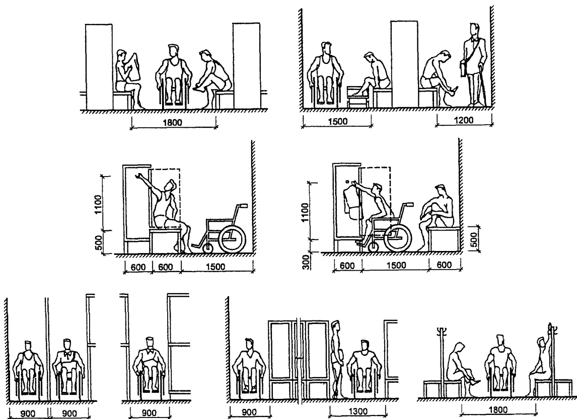
Рис. 5.4. Оборудование ножных ванн и выплыва из душевых в открытый бассейн
