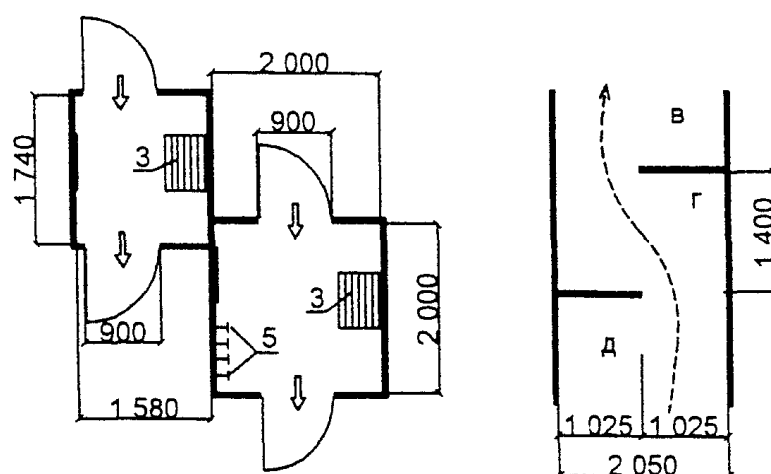
Спортивные индивидуальные кабины для переодевания
