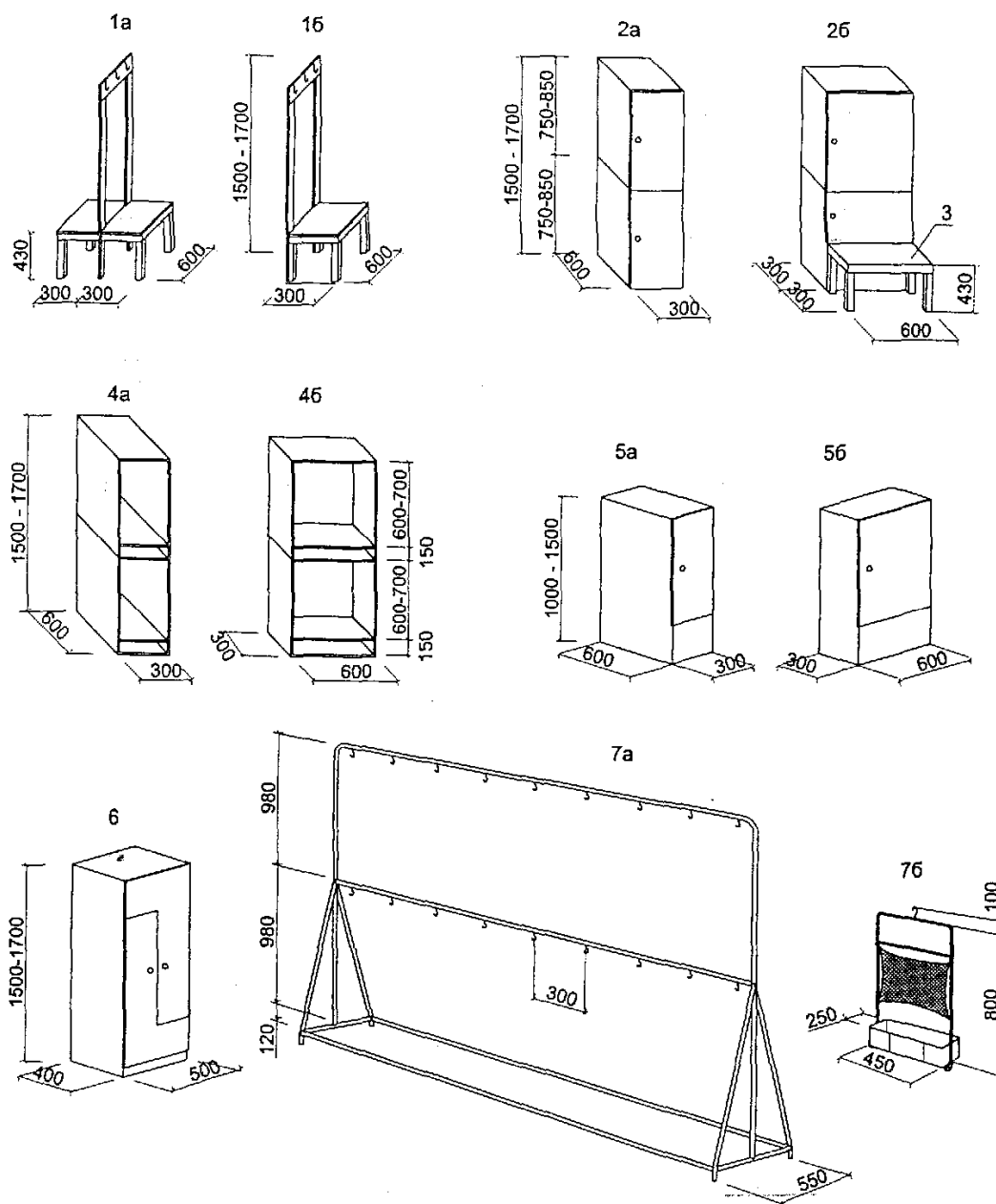
Рис. 5.2. Мебель и оборудование. Габаритные схемы
