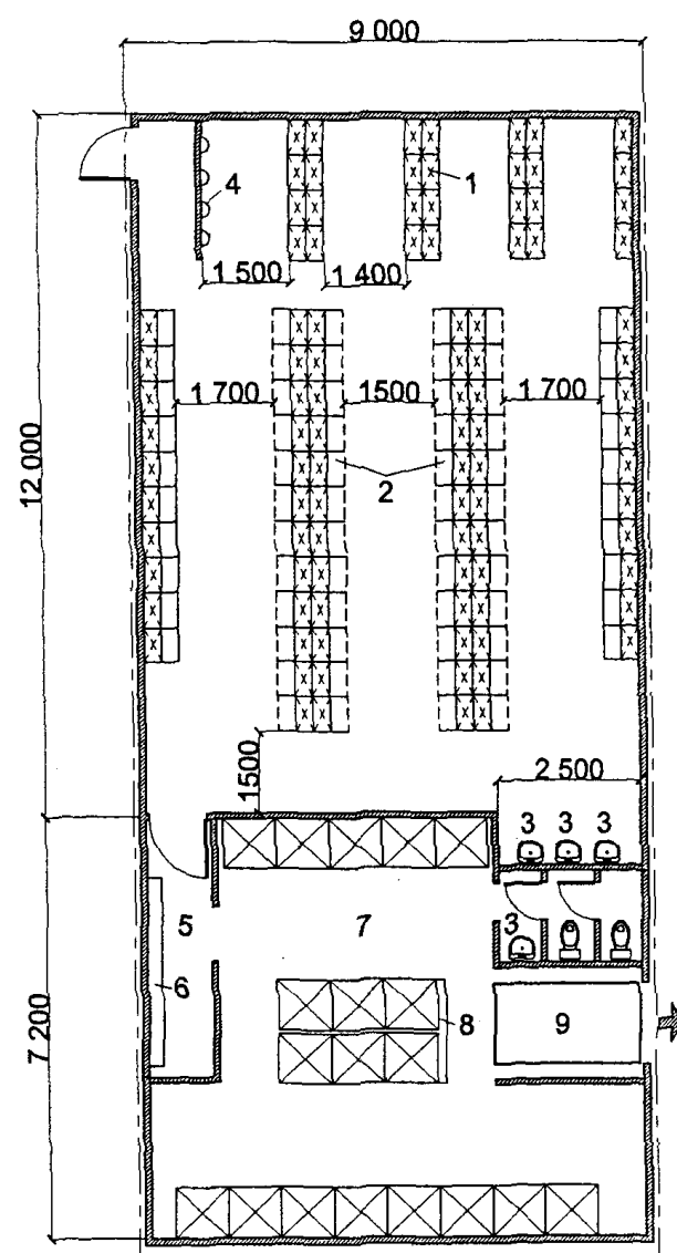
При ванне для плавания 25 x 11 м
