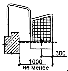
Свободно плавающие ворота
