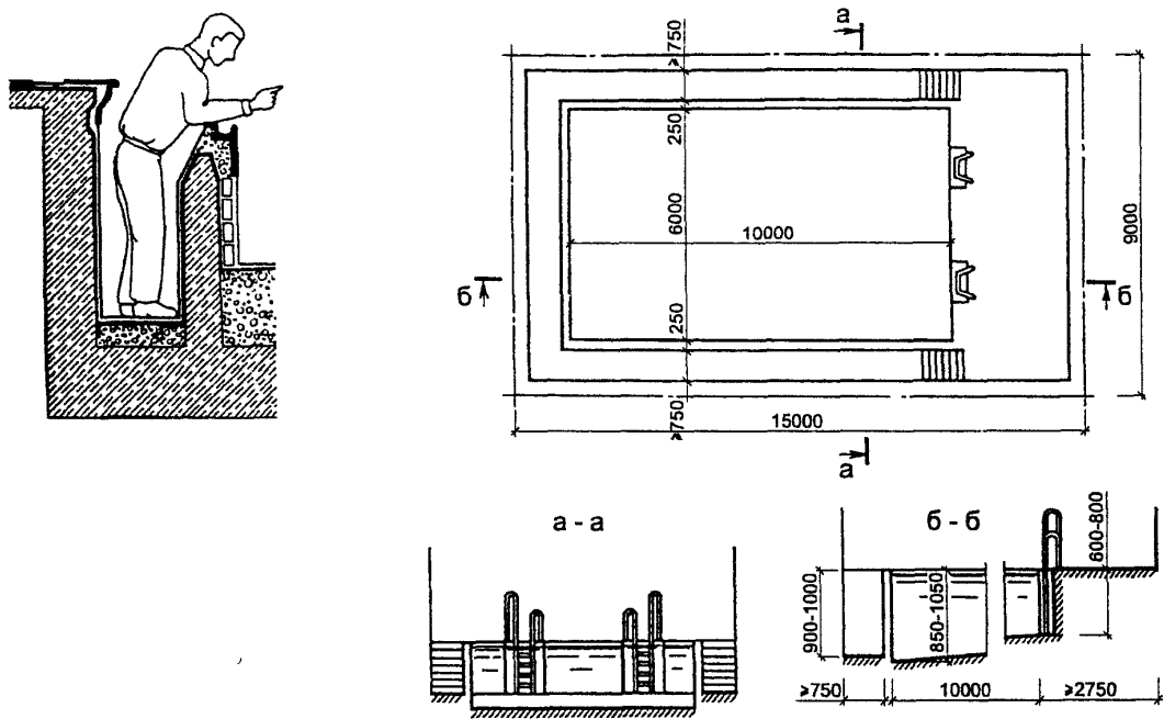
Схема зала бассейна с ванной оздоровительного плавания размером 16,6 x 6,0 м (с учетом обеспечения занятий инвалидов-опорников)
