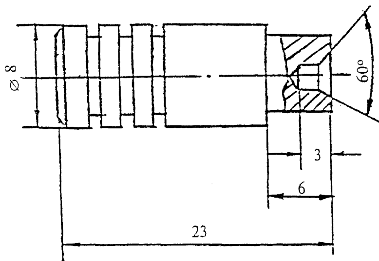
Рисунок 13. Репер для испытаний
