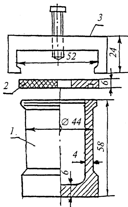
1 - корпус; 2 - крышка; 3 - захват
