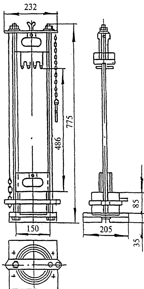
Рисунок 7. Копер ПМ
