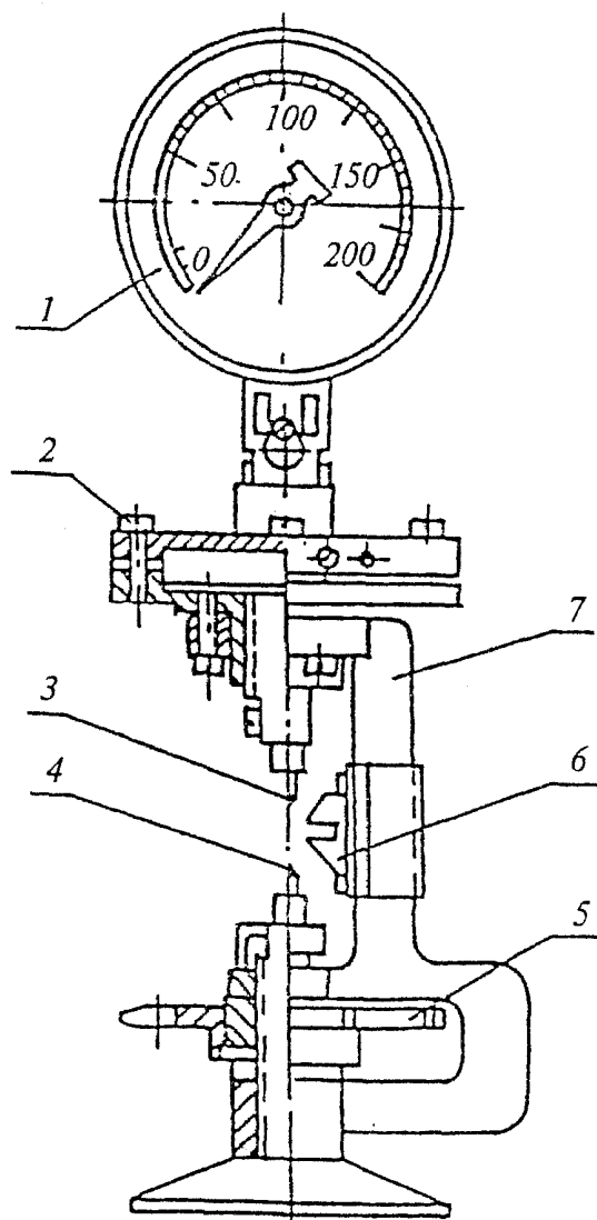
1 - манометр; 2 - гидравлическая мессдоза; 3 - верхний зуб; 4 - нижний зуб; 5 - диск винтового механизма; 6 - щелевой упор; 7 - корпус прибора
