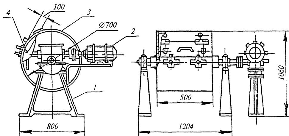
1 - станина; 2 - двигатель; 3 - барабан;
