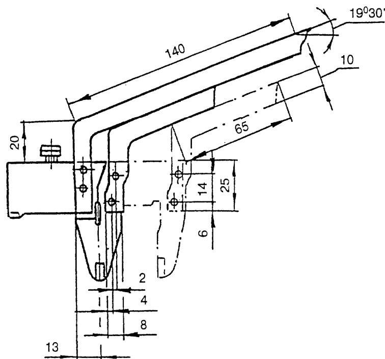
Рисунок 3. Передвижной шаблон
