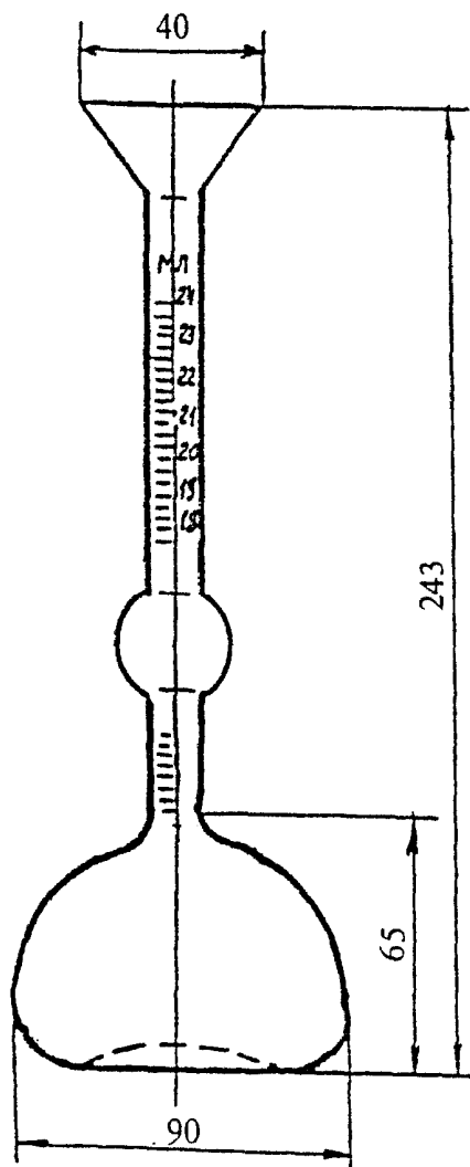
Рисунок 8. Прибор Ле Шателье
