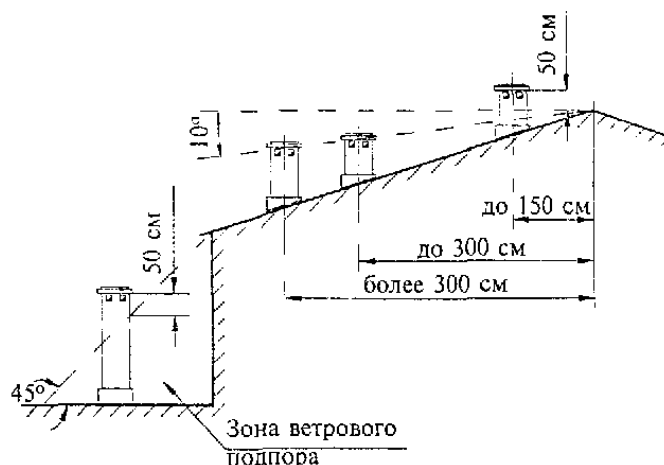
Рисунок 1. Варианты выбора высоты дымохода
