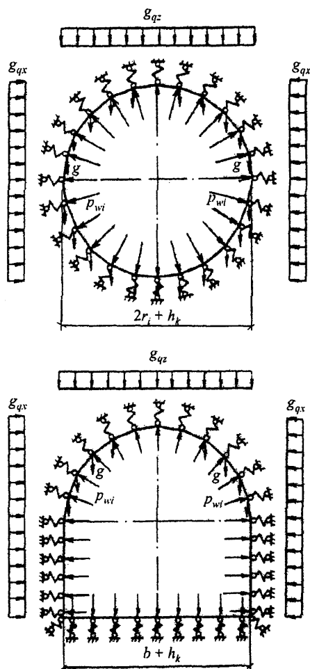
Рисунок А.1. Расчетные схемы обделок туннелей
