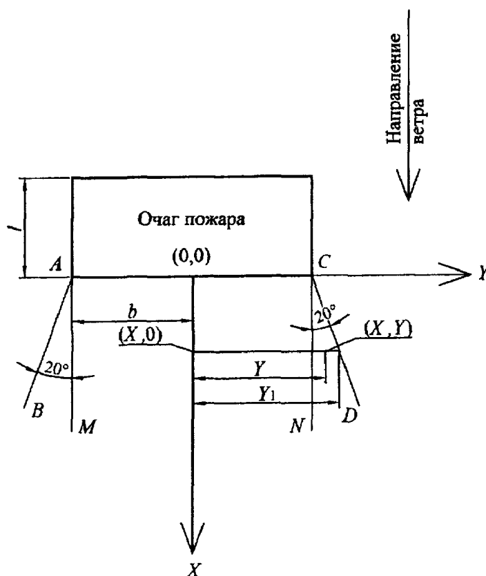
Рисунок Е.1. Схема определения размеров зон загазованности от отдельного очага при направлении ветра перпендикулярно к фасаду здания
