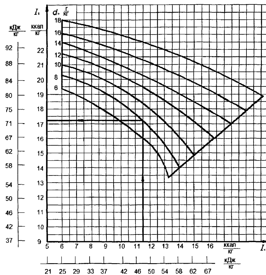
Рисунок Д.1. Определение теплосодержания (энтальпии) внутреннего воздуха при удалении теплоизбытков системой вентиляции в I режиме и допустимых сочетаний температуры и влажности этого воздуха в первой и второй климатических зонах
