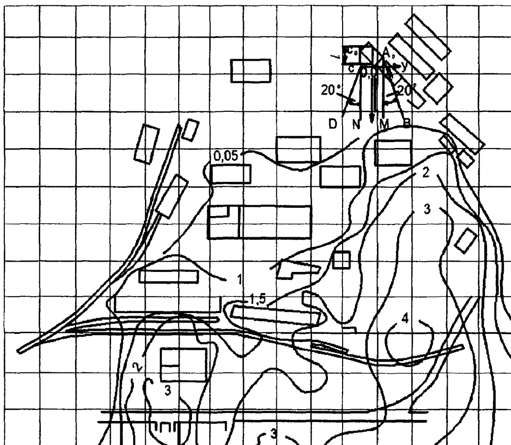
Рисунок Е.3. Схема определения размеров зон загазованности для разных очагов пожара
