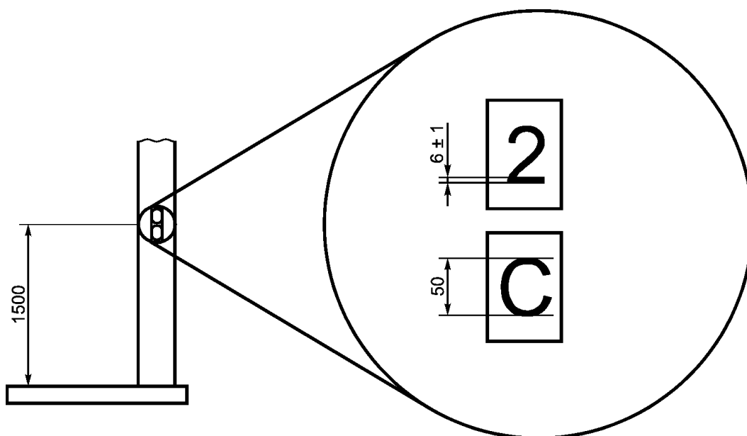
Рисунок А.2 - Размеры символов
