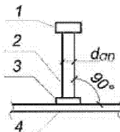
1 - головка анкера; 2 - анкер; 3 - сварка; 4 - стальной опорный элемент
