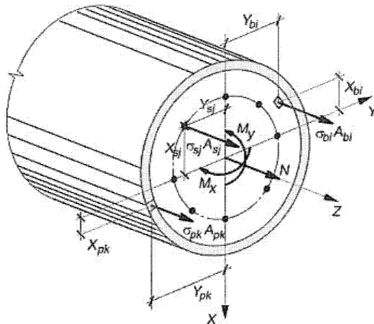
Рисунок 7.4 - Расчетная схема нормального сечения трубобетонного элемента
