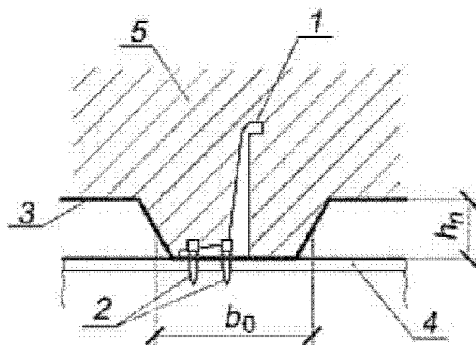
1 - угловой анкер; 2 - дюбель; 3 - настил; 4 - опорная балка; 5 - бетон плиты
