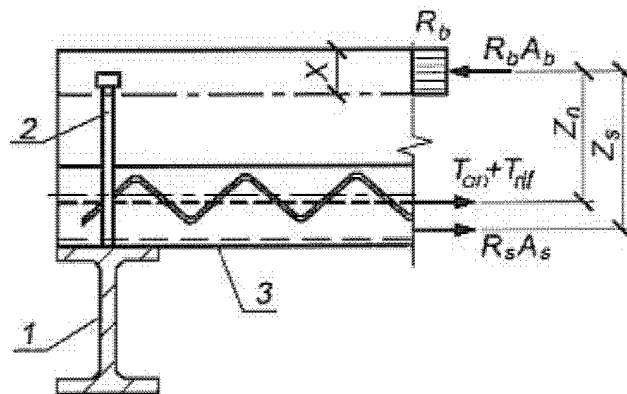
1 - прогон; 2 - анкер; 3 - стальной профилированный настил
