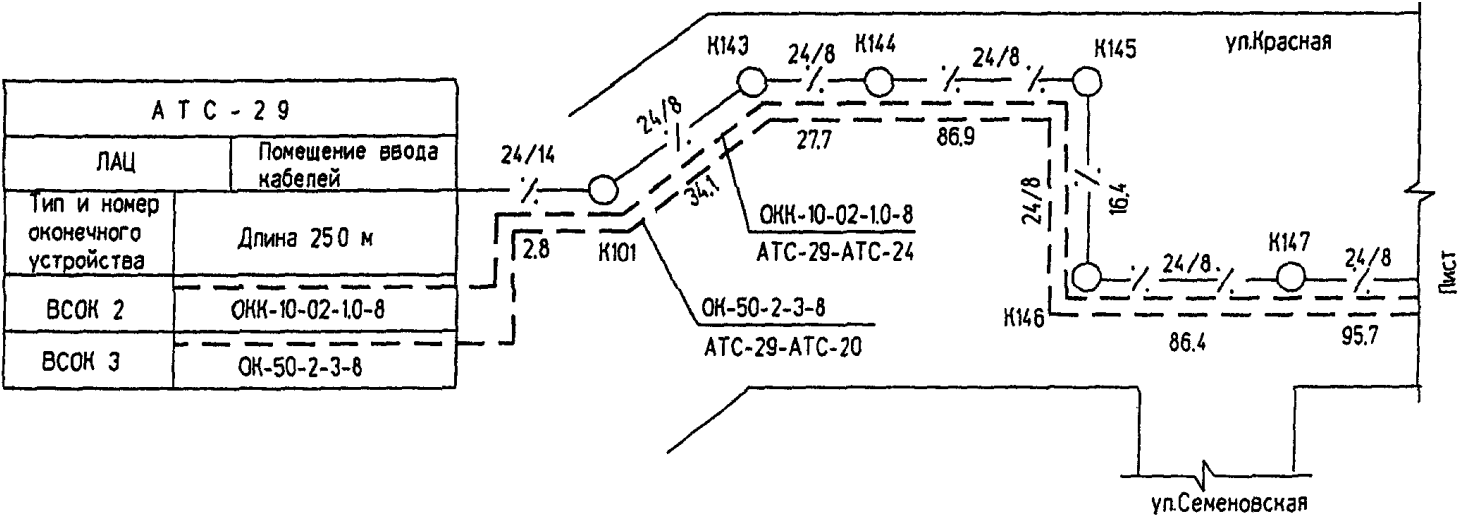
ПРИМЕР ВЫПОЛНЕНИЯ СХЕМЫ РАСПОЛОЖЕНИЯ КАБЕЛЕЙ СВЯЗИ В КАБЕЛЬНОЙ КАНАЛИЗАЦИИ
