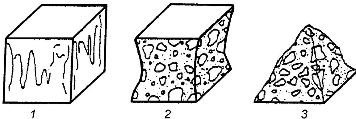
Рисунок Е.1. Удовлетворительные разрушения образцов-кубов
