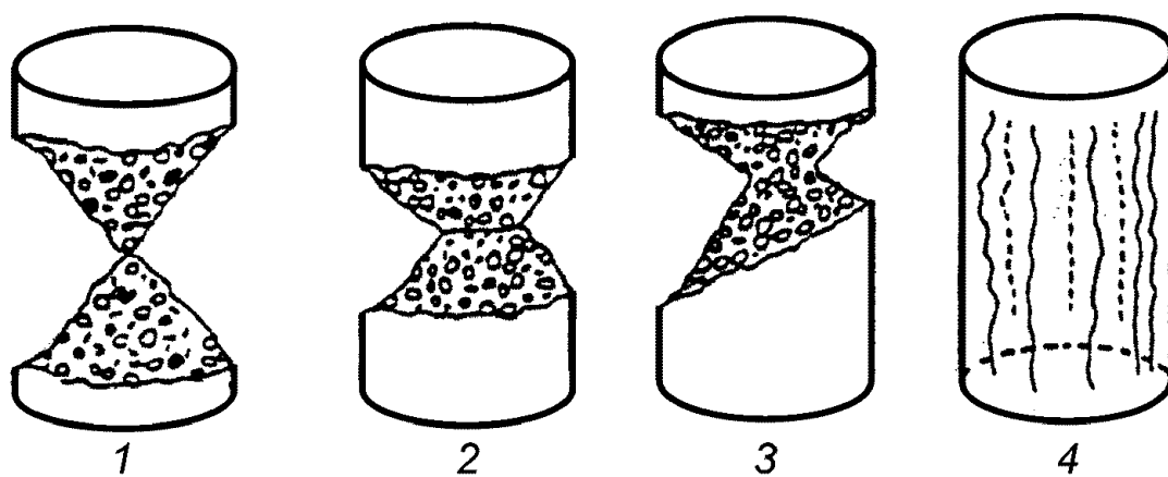
Рисунок Е.3. Удовлетворительные разрушения образцов-цилиндров
