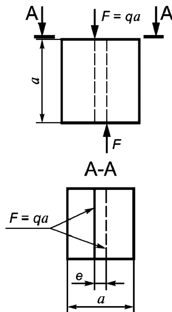
а) С эксцентриситетом
