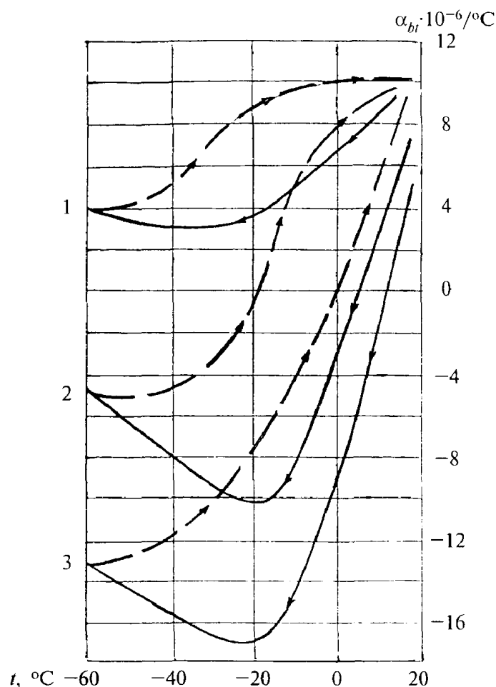
Рисунок 4.2. Коэффициент температурной деформации бетона на портландцементе с силикатным заполнителем
