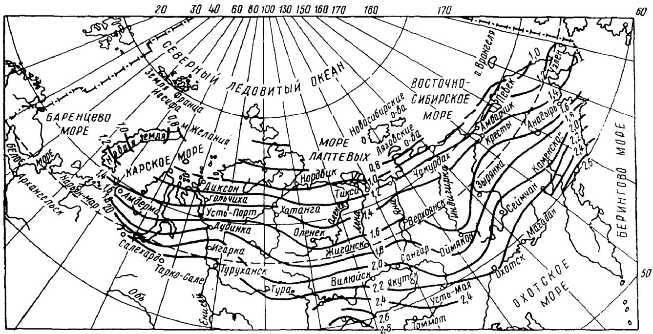
Изолинии глубин сезонного оттаивания песчаных грунтов
