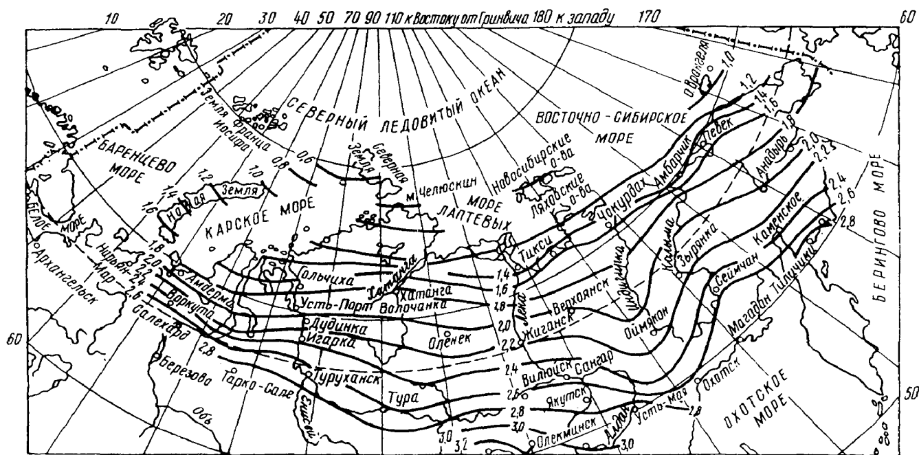
Изолинии глубин сезонного оттаивания заторфованных грунтов
