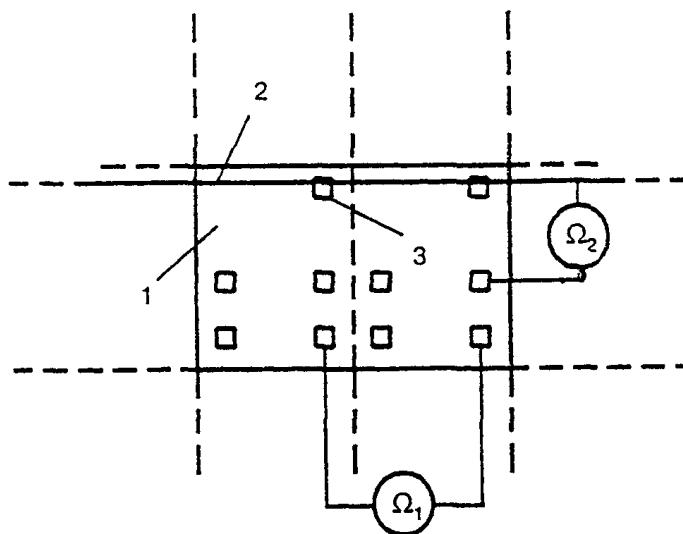
1 - блок; 2 - шина заземления; 3 - закладные детали
