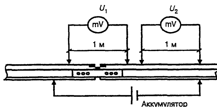
Рисунок 3. Схема измерения сопротивления сборного стыка ходового рельса двумя милливольтметрами
