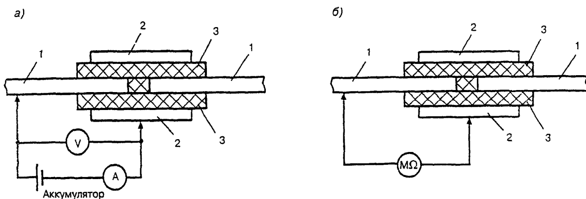
1 - рельс; 2 - путевая накладка; 3 - изолирующие конструктивные элементы
