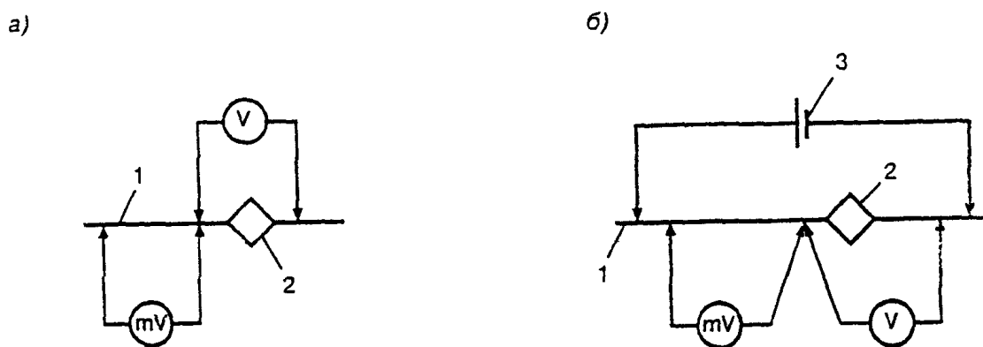
1 - кабель; 2 - изолирующая муфта; 3 - источник тока
