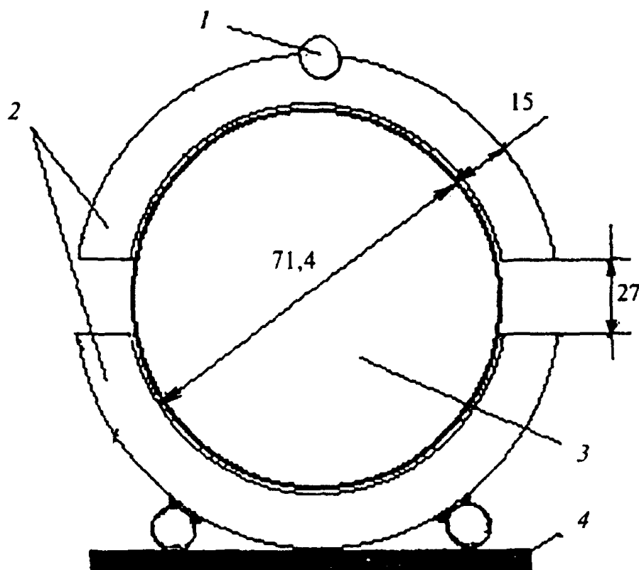
1 - шарнир; 2 - цилиндрические обоймы; 3 - образец; 4 - нижняя плита прессы
