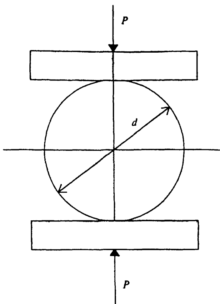
Рисунок 7. Схема испытания образцов на растяжение при расколе
