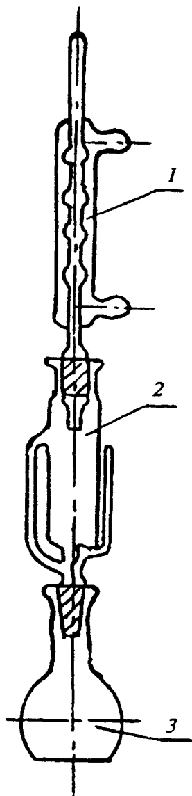
Рисунок 11. Аппарат типа Сокслет
