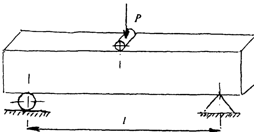
Рисунок 8. Схема испытания образцов-призм на изгиб
