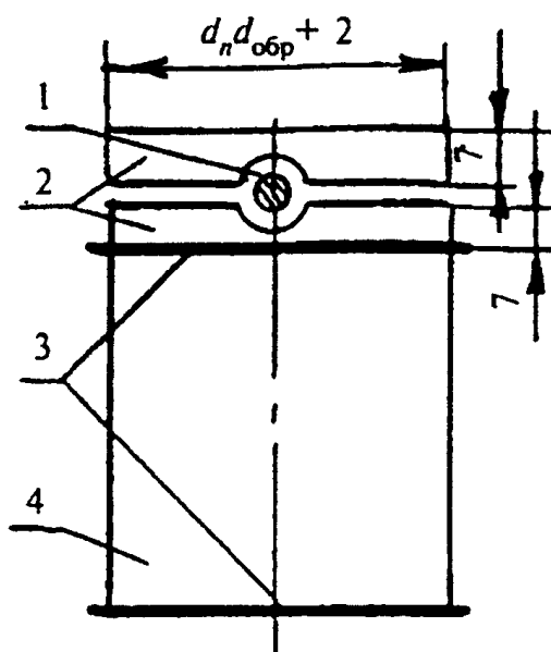
Рисунок 6. Шарнирное устройство
