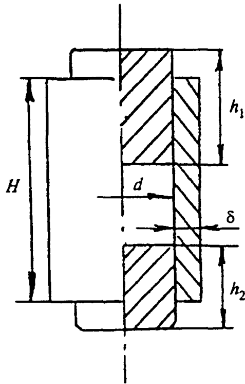
Рисунок 1. Форма одиночная обычная
