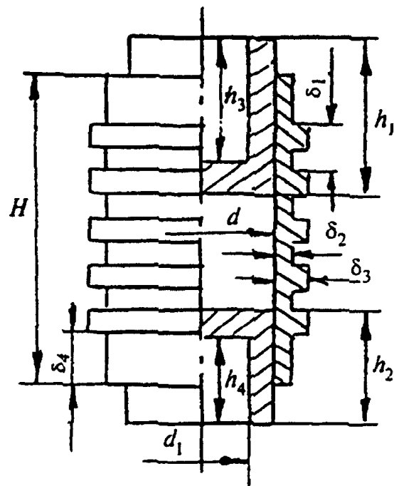
Рисунок 2. Форма одиночная облегченная
