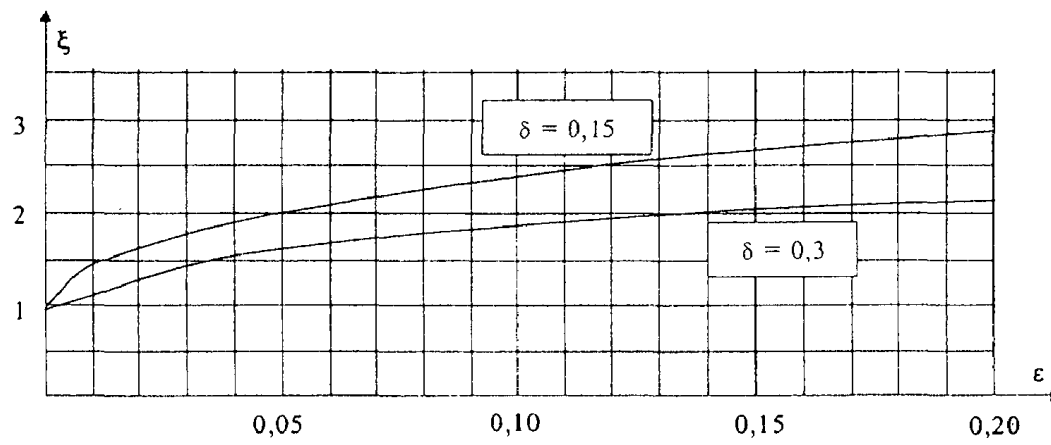
Рисунок 11.1. Коэффициенты динамичности
