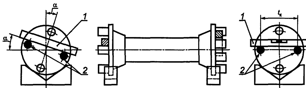
1 - пузырьковый уровень; 2 - центровочный штырь
