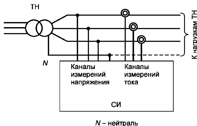
Рисунок Б.8. Схема измерений мощности
