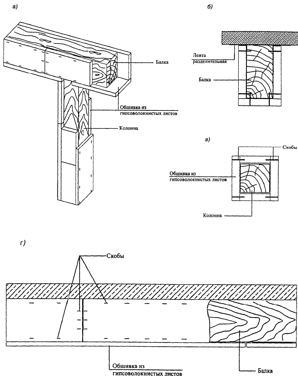
Рисунок 16. Общий вид (а), конструктивное решение огнестойкости деревянной балки (б, г) и колонны (в)
