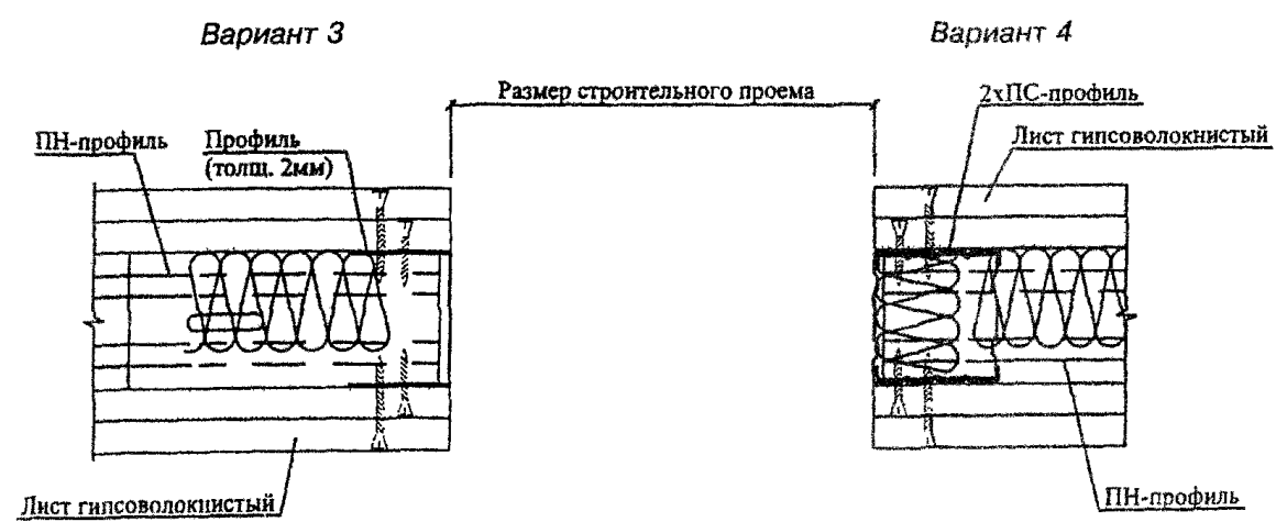
Рисунок 4. Температурные швы и варианты дверных проемов в перегородках
