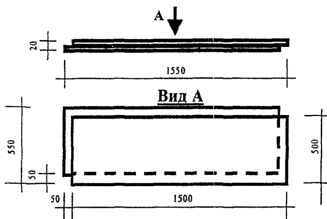
Рисунок 14. Элемент сборного основания пола
