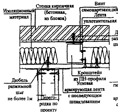
Б Т-сопряжение
