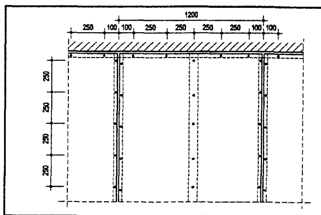
Рисунок 18. Крепление гипсоволокнистых листов к каркасу
