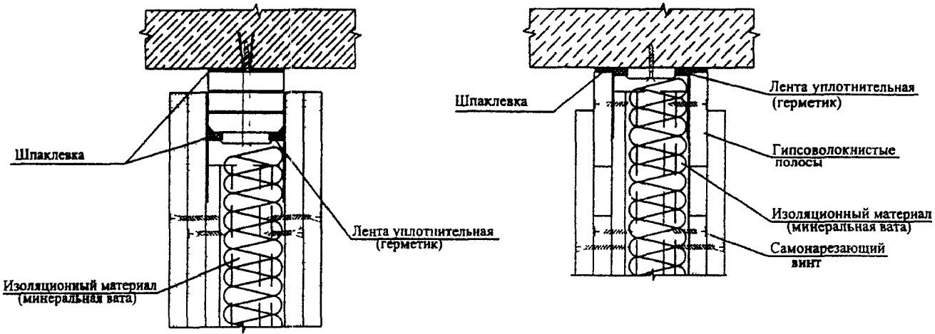
Подвижное присоединение, связанное с замкнутой системой подвесного потолка
