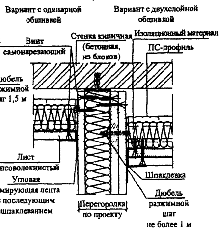
В Т-сопряжение
