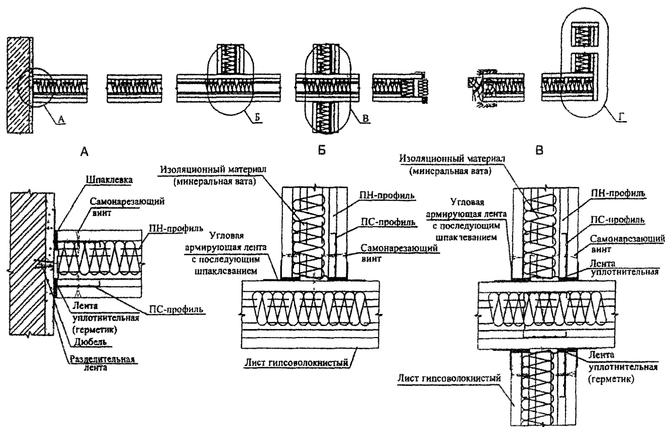
Вертикальный разрез
