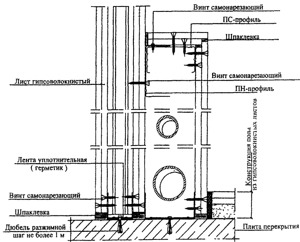
Рисунок 10. Конструктивное решение оформления трубопроводов, размещенных вдоль капитальной стены (а), перегородки (б)
