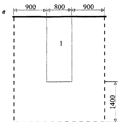
а - четырехместная жилая комната; б - шестиместная жилая комната; в - зона размещения кровати для лиц, способных к частичному самообслуживанию и передвигающихся по дому
