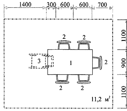
Место для питания на 6 чел.
