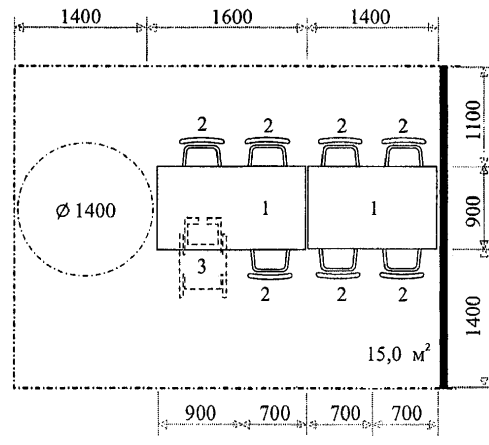
Место для питания на 8 чел.
