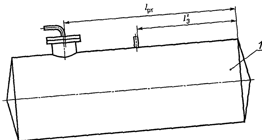
Рисунок А.11. Схема резервуара с расходной трубой (рисунок А.11 введен Изменением N 1 , введенным в действие Приказом Росстандарта от 17.09.2012 N 308-ст)
