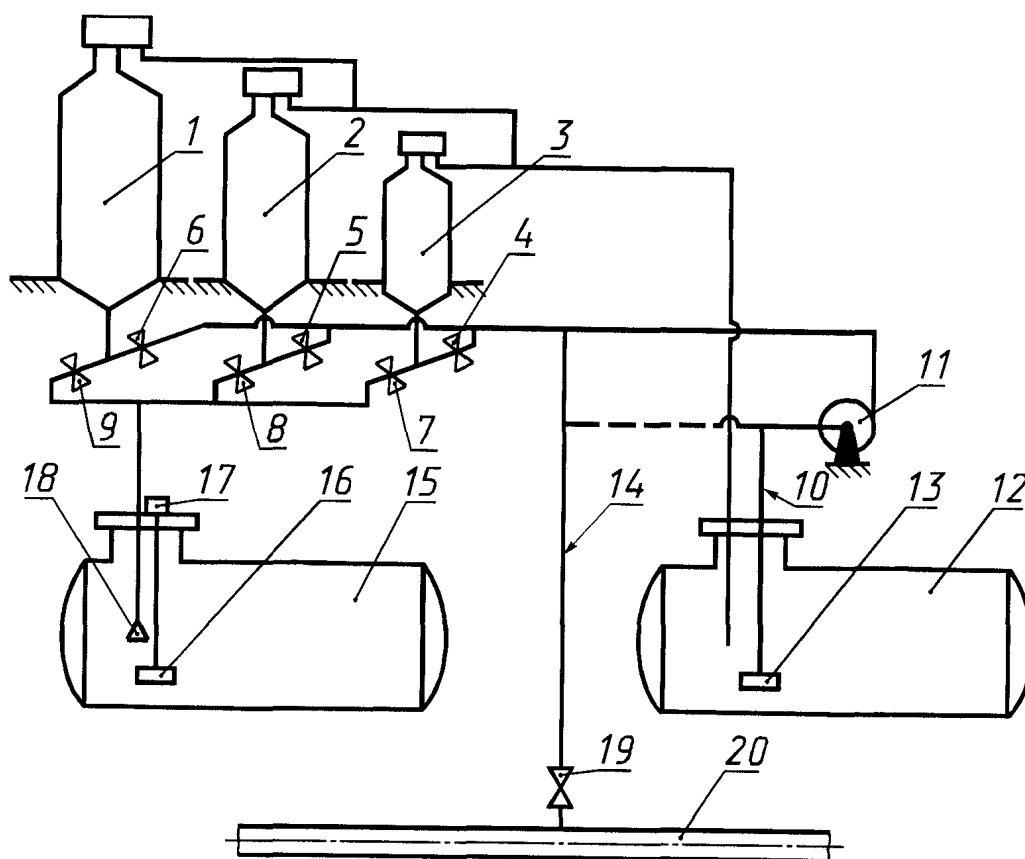
1, 2, 3 - мерники; 4, 5, 6 - вентили наполнения; 7, 8, 9 - вентили опорожнения; 10 - всасывающая линия насоса; 11 - насос; 12 - приемный резервуар; 13 - фильтр; 14 - линия технологической обвязки; 15 - поверяемый резервуар; 16 - поплавок уровнемера; 17 - уровнемер; 18 - расширитель струи; 19 - вентиль обвязки; 20 - технологический трубопровод (водопровод)
