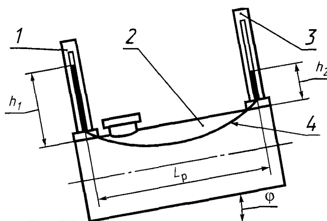
1, 3 - водомерные трубки; 2 - резервуар; 4 - резиновая трубка
