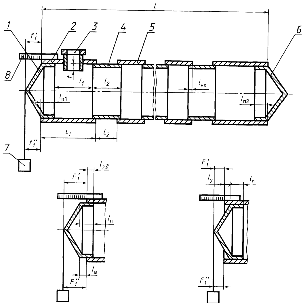
Рисунок А.1. Схема двойного отвеса
