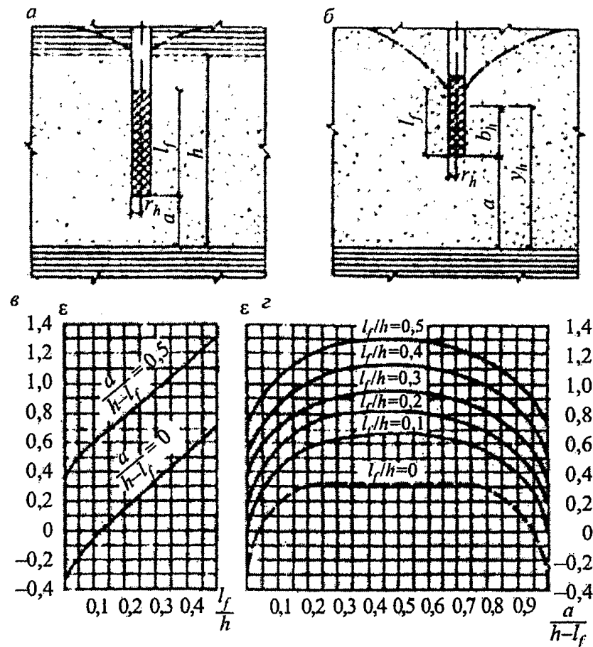
а, б - схемы несовершенных скважин в напорном и безнапорном пластах; в, г - графики для определения \varepsilon
