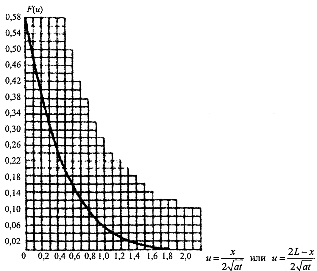
Рисунок А.1. График функции F(u)
