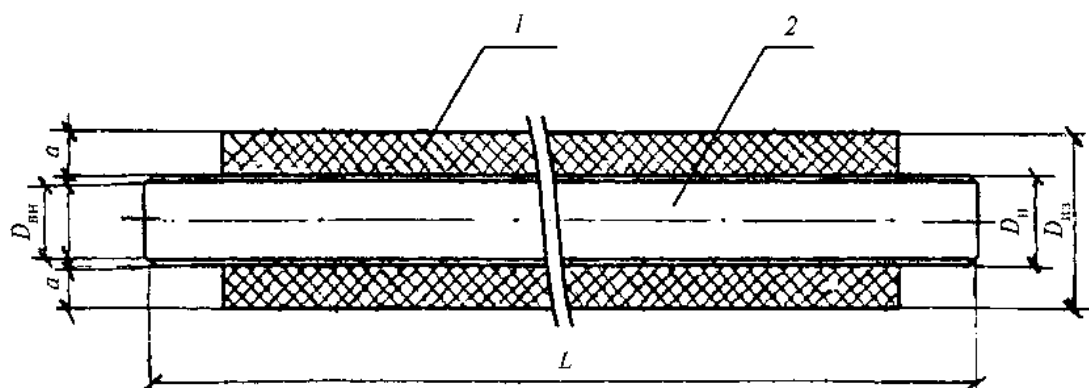
1 - изоляция из ППМ; 2 - асбестоцементная труба; D_{\text{вн}} - внутренний диаметр трубы; D_{\text{н}} - наружный диаметр трубы; D_{\text{из}} - внешний диаметр изоляции; L - длина трубы; а - толщина изоляции
