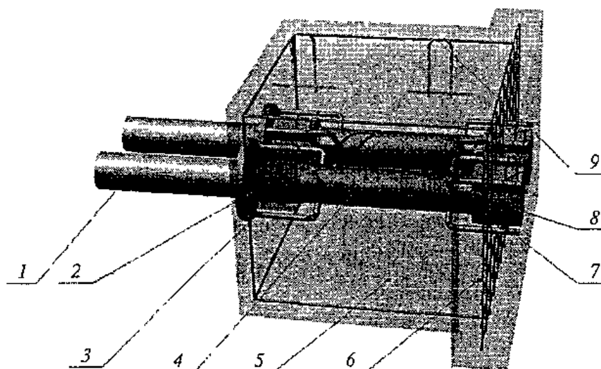
Рисунок 1. Узел ответвления стального трубопровода D_y = 150 мм налево от асбестоцементного D_y = 200 мм
