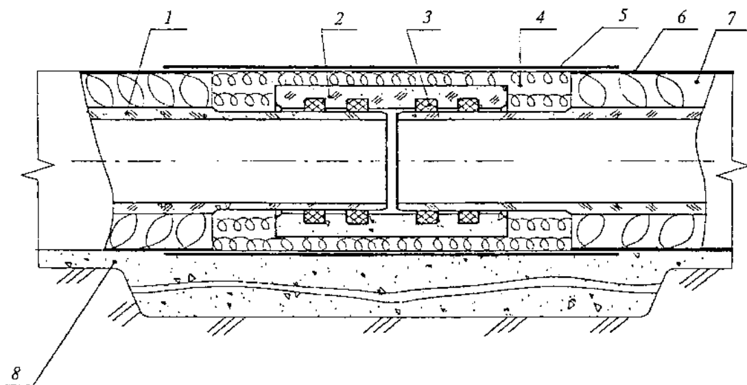
1 - асбестоцементная труба; 2 - асбестоцементная муфта; 3 - резиновые уплотнительные кольца; 4 - полуцилиндры (сегменты) из ППУ; 5 - термоусаживающаяся полиэтиленовая муфта; 6 - полиэтиленовая оболочка теплоизоляции; 7 - теплоизоляция из ППУ; 8 - слой песка
