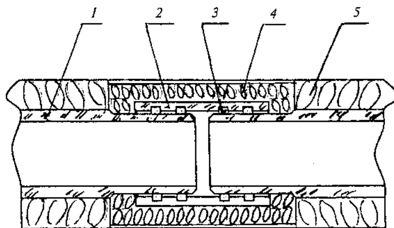
1 - асбестоцементная труба; 2 - асбестоцементная муфта; 3 - резиновые уплотнительные кольца; 4 - изоляция стыка из ППМ; 5 - теплоизоляция из ППМ
