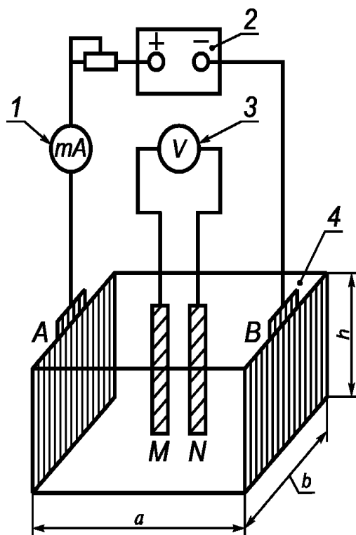
1 - миллиамперметр; 2 - источник тока; 3 - вольтметр; 4 - измерительная ячейка размерами a , b ; h (см. A.2.2); A и B - внешние электроды; M и N - внутренние электроды
