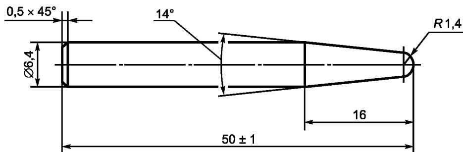
Рисунок Ф.2 - Размеры резца для выполнения прорезания
