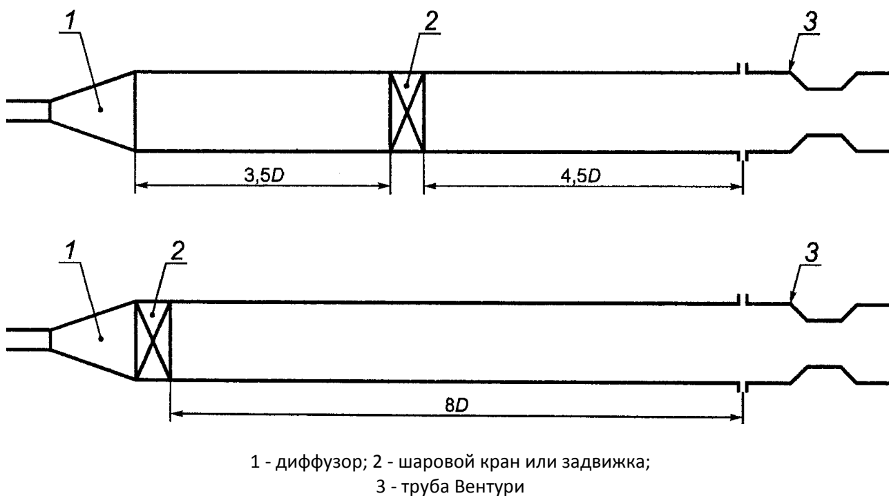
Рисунок 2. Схема расположения шарового крана или задвижки при \beta = 0,6
