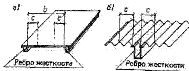
а - плоский лист; б - гофрированный лист
