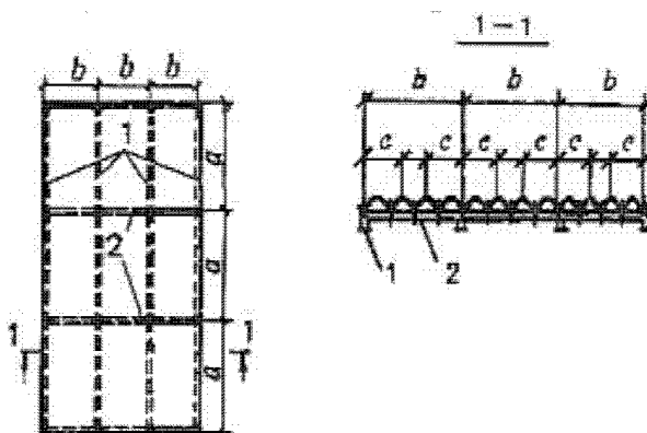
1 - продольные ребра; 2 - поперечные ребра
