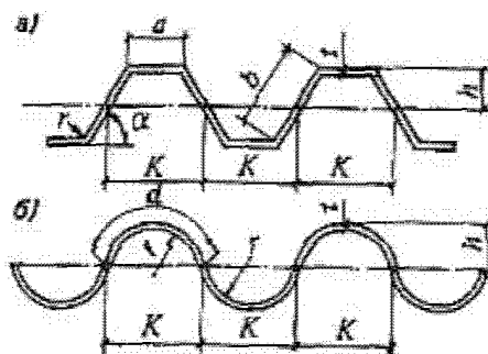
а - трапециевидный гофр; б - волнистый гофр
