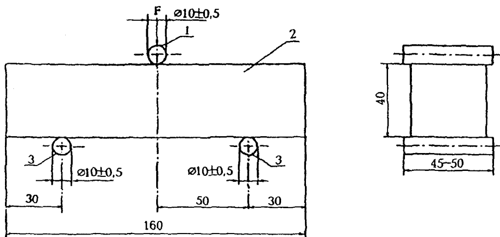
1 - нагрузочный элемент; 2 - образец-балочка; 3 - опора
