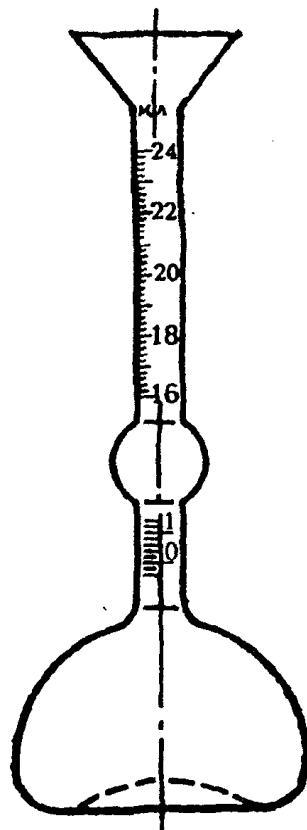
Рисунок 1. Прибор Ле Шателье
