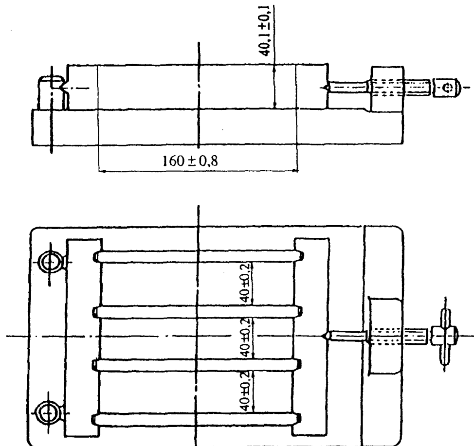
Рисунок 8. Форма для изготовления образцов-балочек
