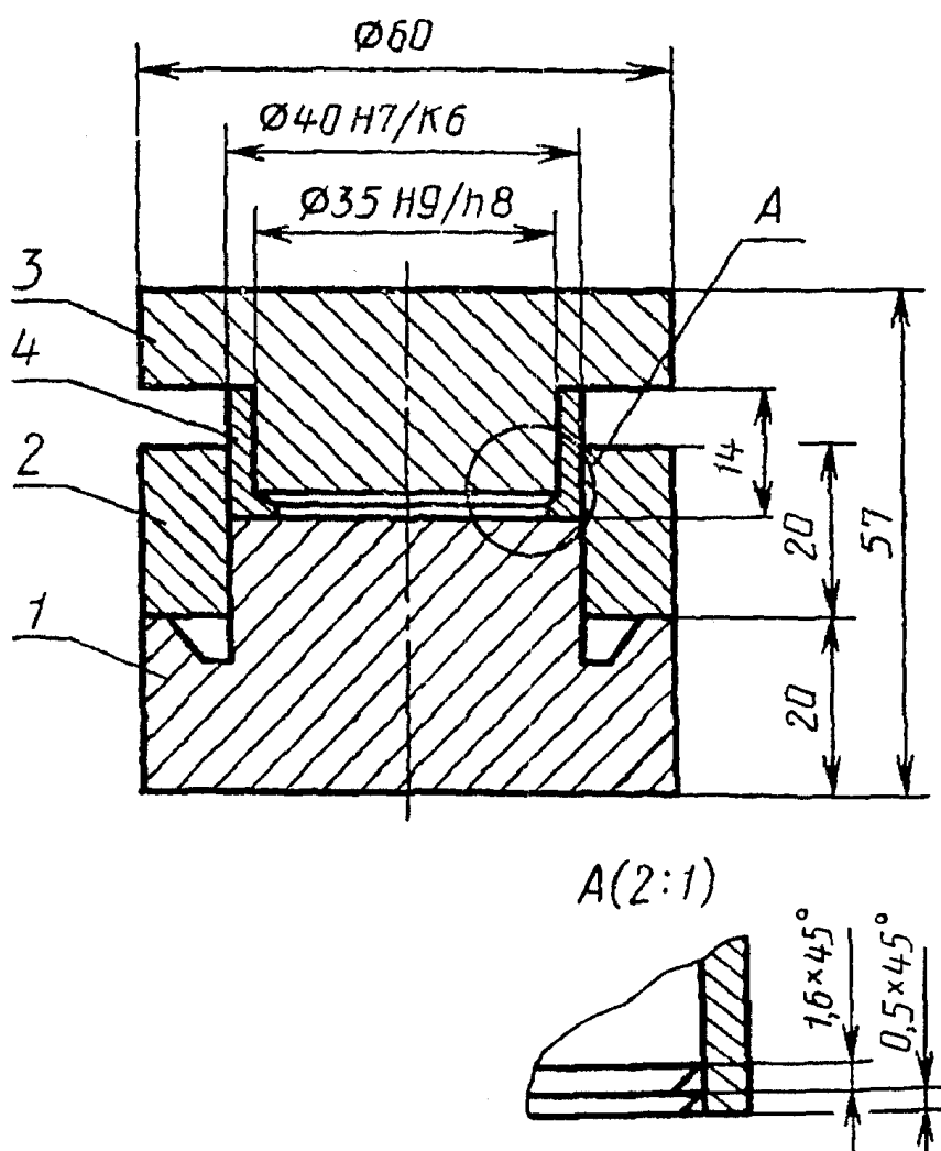
Пресс-форма
