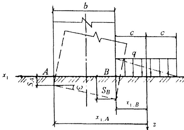
Рисунок 2. Схема к определению крена сооружения от пригрузки
