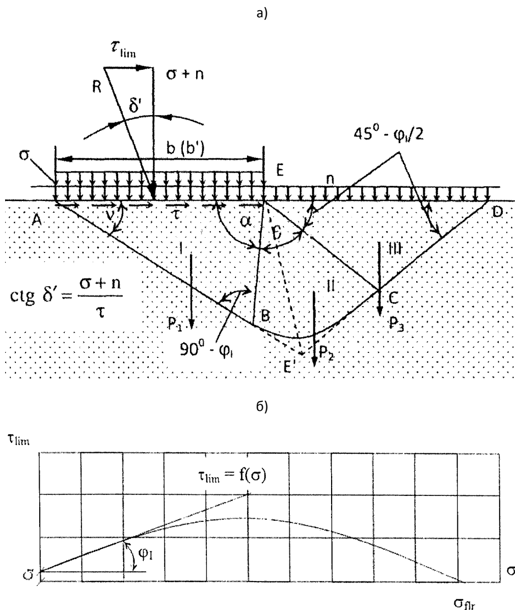
а - расчетная схема; б - график несущей способности основания; I, II, III - зоны призмы обрушения
