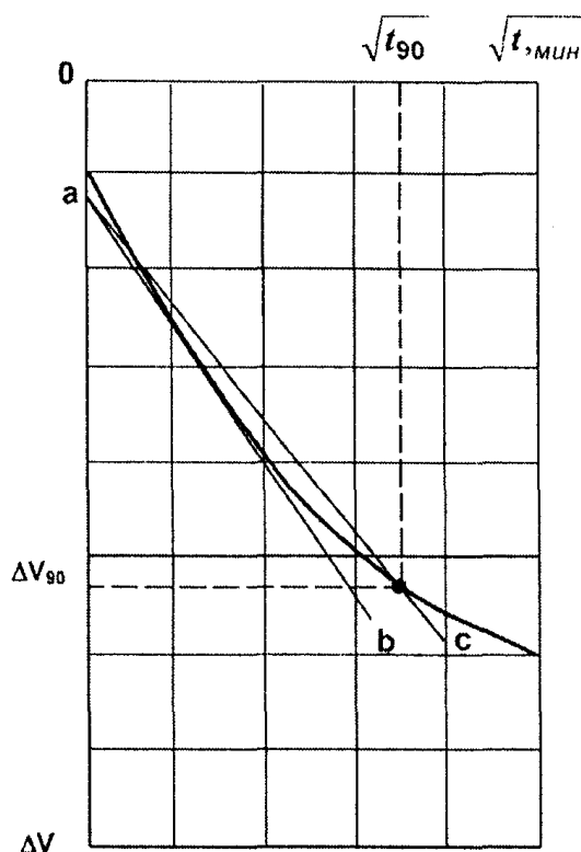
Рисунок Б.1. Графический способ определения 90% первичной консолидации методом "квадратный корень из времени"
