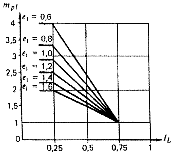
Рисунок В.1. График для определения коэффициента m_{pl}
