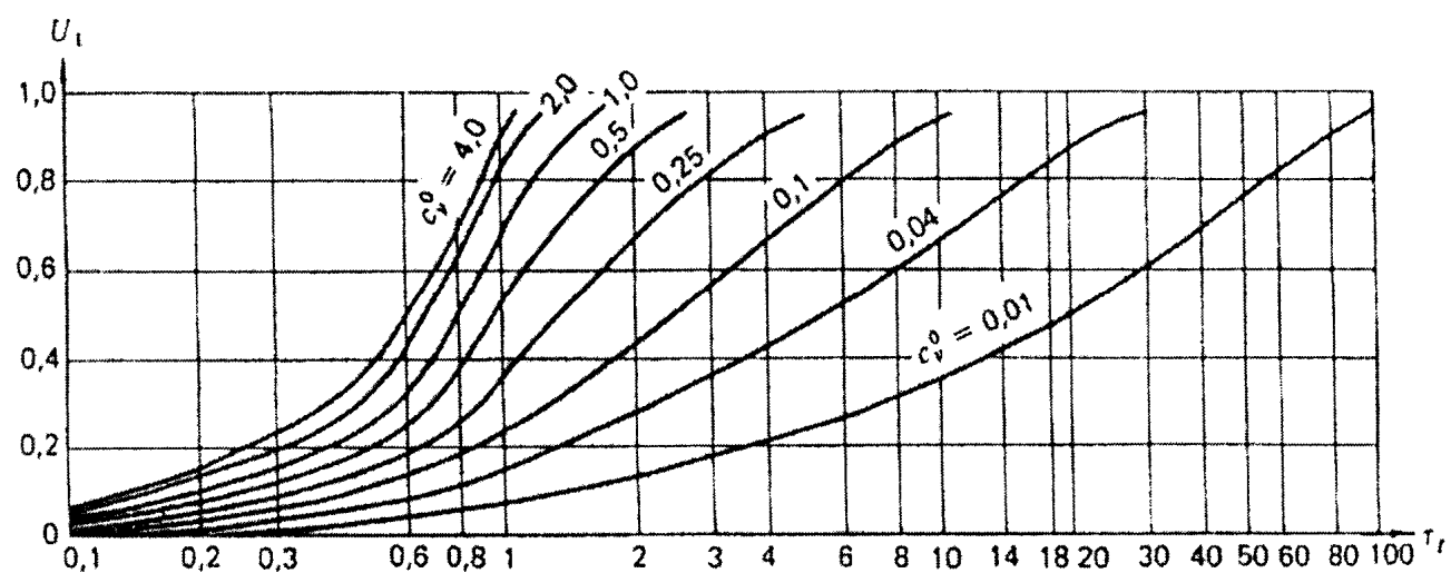
Рисунок М.1. График зависимости степени консолидации U_1
