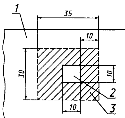
1 - испытуемое покрытие; 2 - образец покрытия сдвига; 3 - расчищенная площадка.
