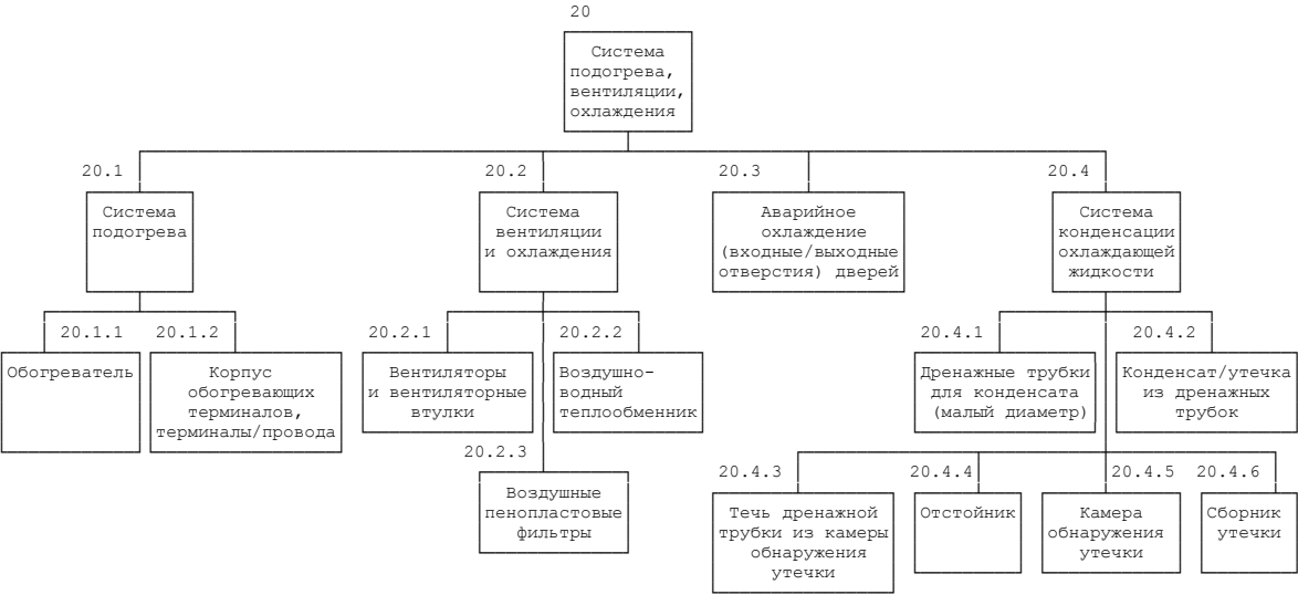
Рисунок В.3. Диаграмма системы нагревания, вентиляции, охлаждения
