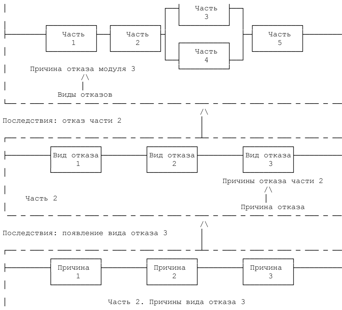
Рисунок 1. Взаимосвязь видов и последствий отказов в иерархической структуре системы
