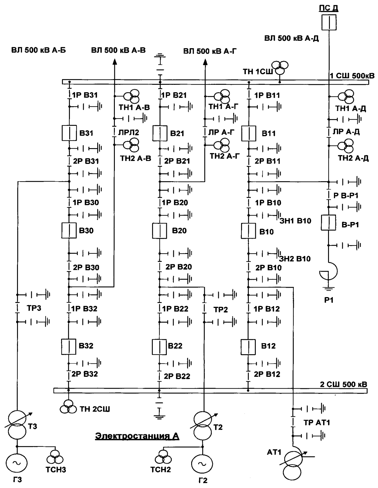
Рисунок 4. Полупотурная схема РУ
