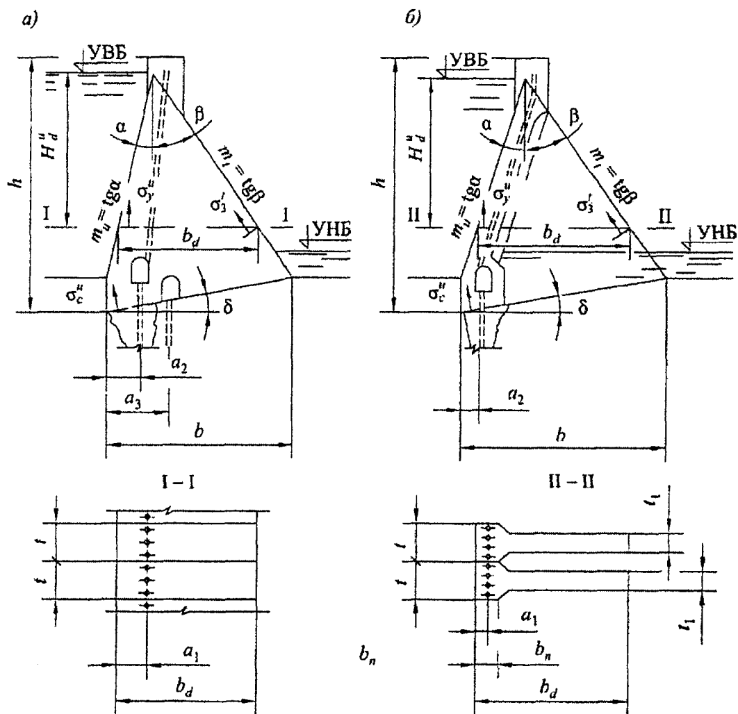
а - массивной; б - с расширенными швами и контрфорсной; h - напор над контактным сечением у верховой грани со стороны верхнего бьефа (высота плотины); b - ширина плотины по основанию; b_d - длина секции; t - длина секции; t_1 - толщина секции в пределах расширенных швов (толщина контрфорса); b_h - толщина торцевого сечения оголовка; a_1 - расстояние от дренажа тела плотины до верховой грани; a_2 - расстояние от оси цементационной завесы до верховой грани; a_3 - расстояние от дренажа основания до верховой грани; H_d^u - напор над расчетным сечением; b_d - ширина расчетного сечения; m_u , m_t - наклоны верховой и низовой граней плотины; \sigma_y^u , \sigma_c^u - нормальные напряжения по горизонтальным площадкам у верховой грани и по площадкам контактного сечения плотины с основанием у верховой грани; \sigma_3^f - максимальные сжимающие главные напряжения у низовой грани плотины
