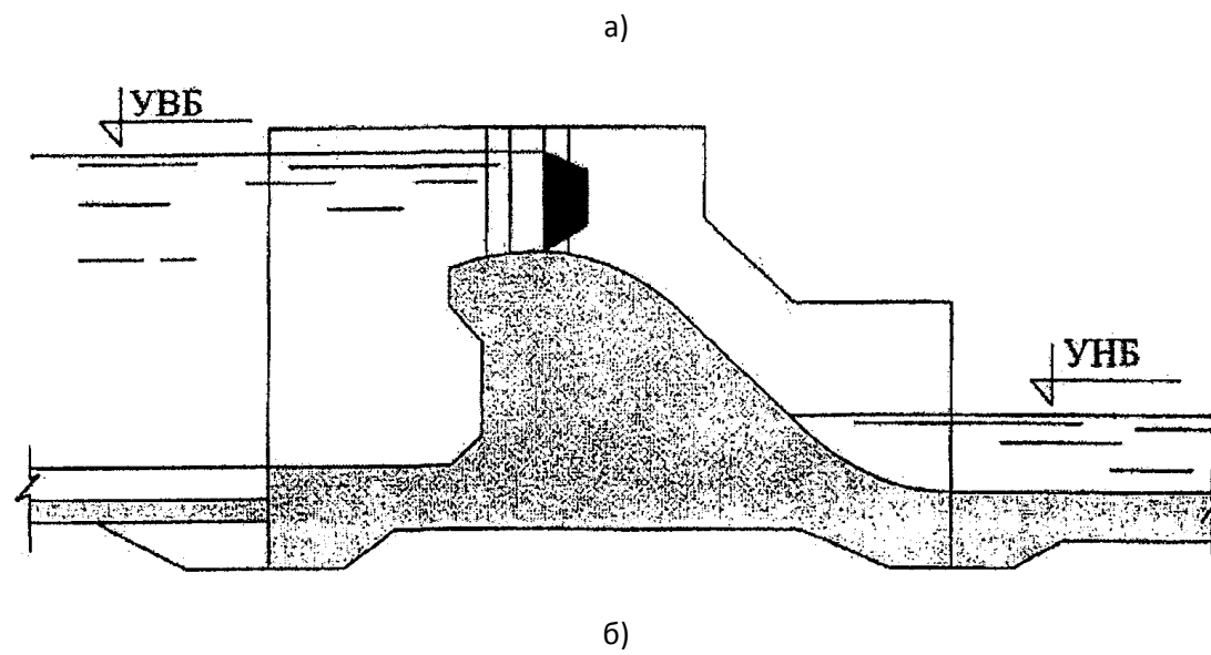
Рисунок 1. Основные виды плотин на скальных основаниях
