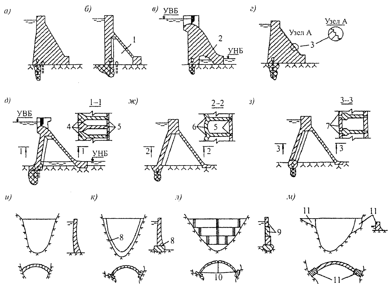
Гравитационные: а - массивные; б - с расширенными швами; в - с продольной полостью у основания; г - со ступенчатой низовой гранью Контрфорсные: д - массивно-контрфорсные; ж - многоарочные; з - с плоским перекрытием
