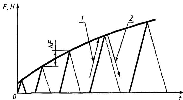
Рисунок 11. Проведение испытаний при ступенчатом увеличении нагрузки 1 - нагрузка; 2 - разгрузка
