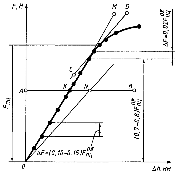
Рисунок 4. Диаграмма испытаний для определения предела пропорциональности при сжатии
