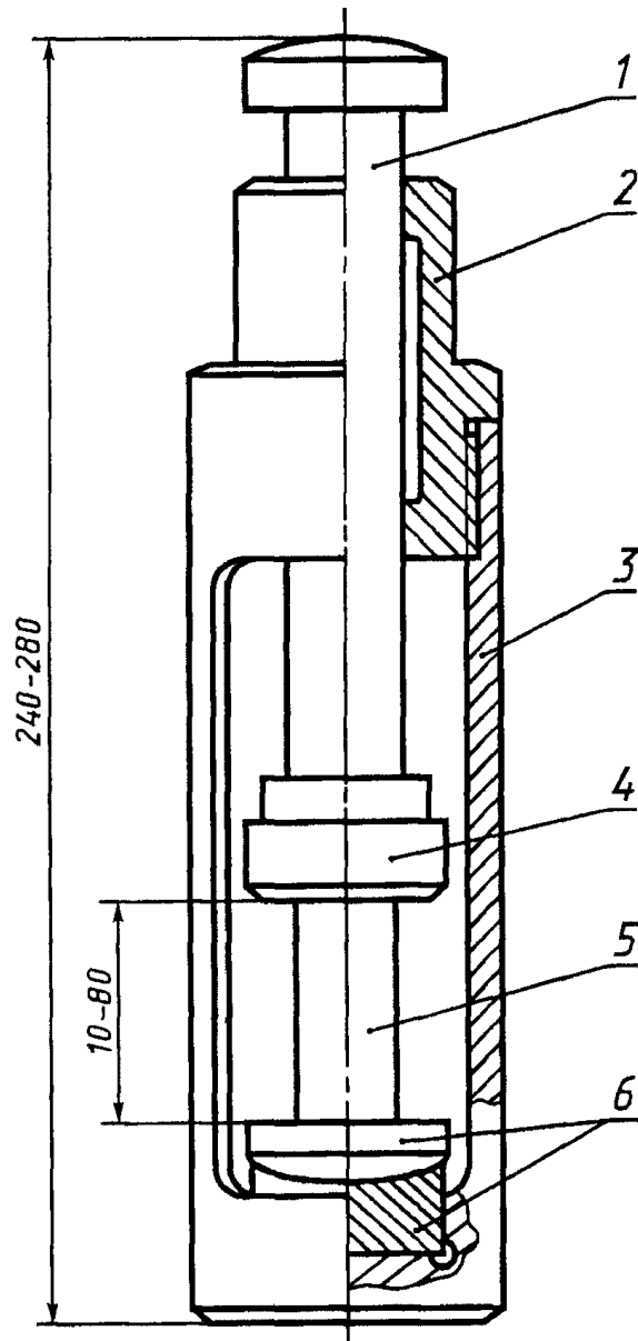
Рисунок В.1. Приспособление для испытания на сжатие: 1 - пуансон; 2 - направляющая втулка; 3 - основание; 4 - опорная верхняя плита; 5 - образец; 6 - самоустанавливающая опора со сменным вкладышем
