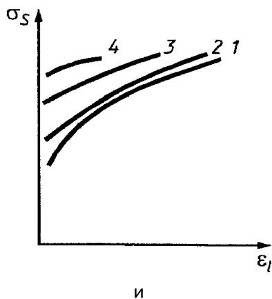
Рисунок Б.1. Типы кривых упрочнения
