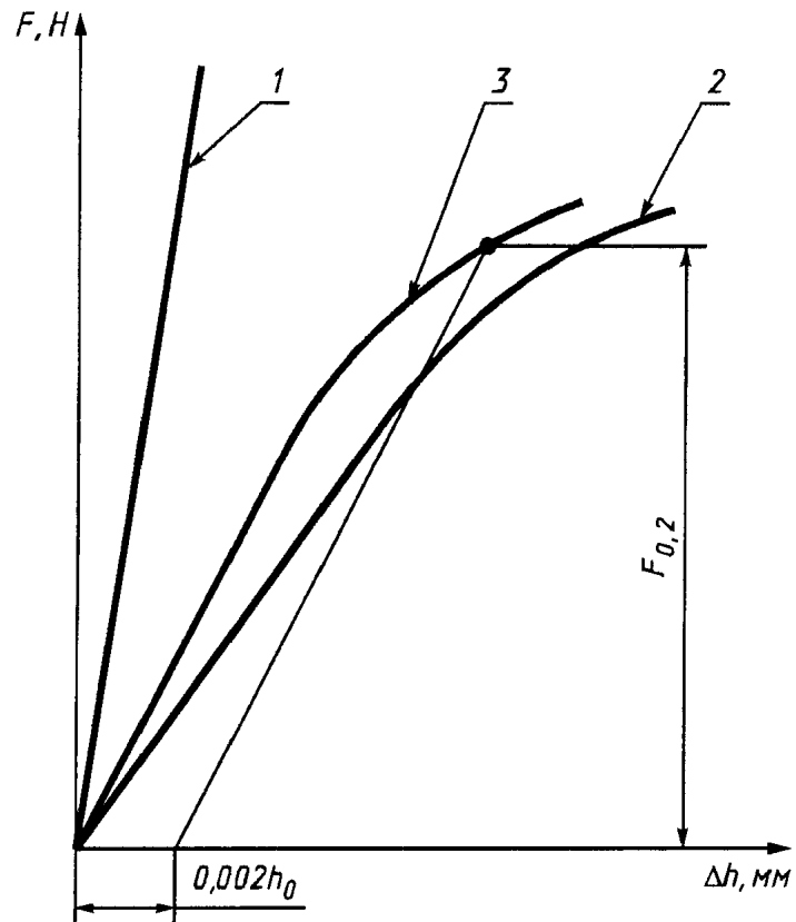
Рисунок 7. Диаграмма испытаний для определения условного предела текучести при сжатии
