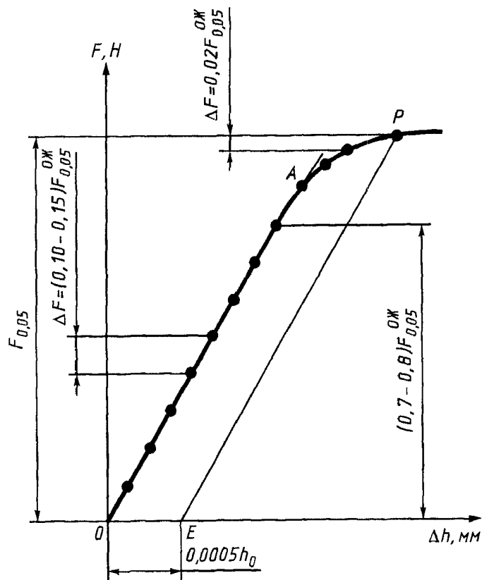
Рисунок 5. Диаграмма испытаний для определения предела упругости при сжатии
