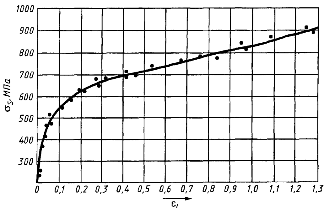
Рисунок 9. Экспериментальная кривая упрочнения в координатах
