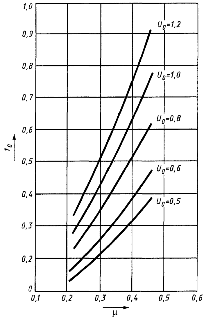
Рисунок А.1. Зависимость оптимального значения высоты буртиков от коэффициента Пуассона
