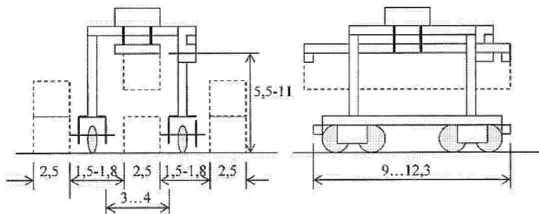
Рисунок 3 - Портальный автопогрузчик
