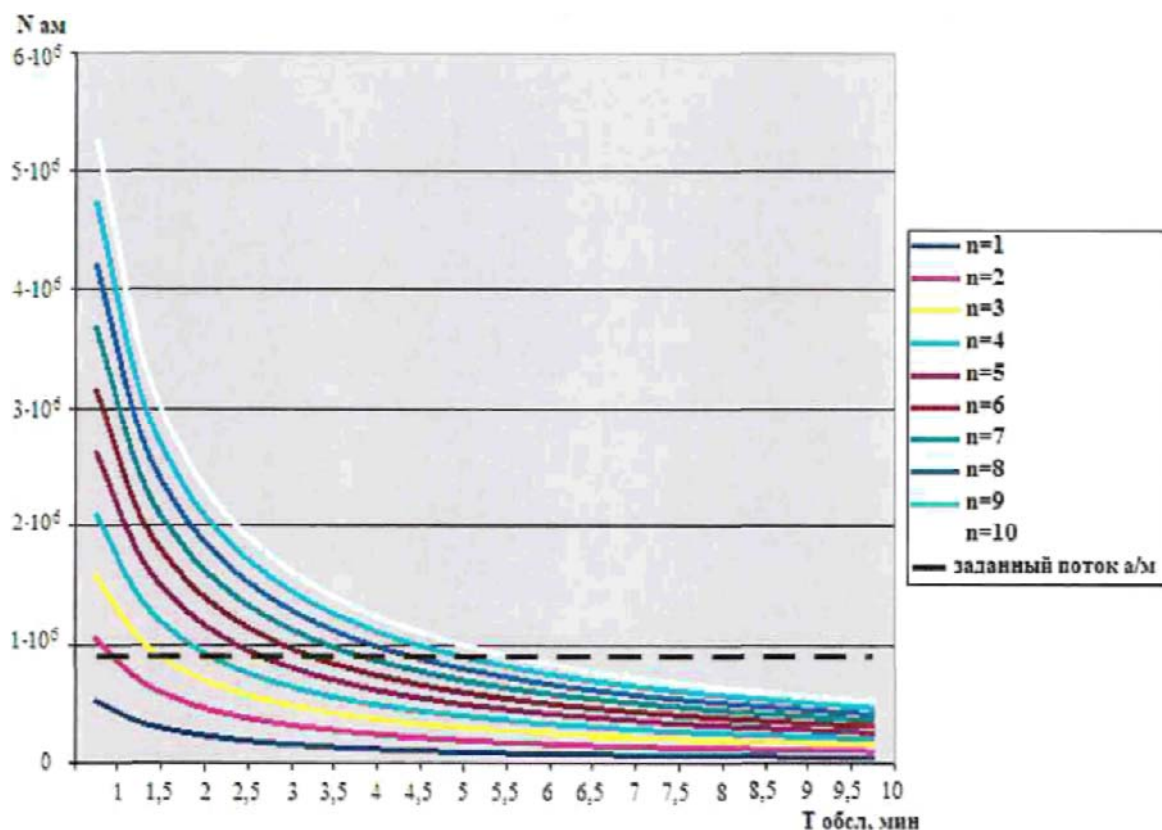
Рисунок Б.1 - Пропускная способность АВК
