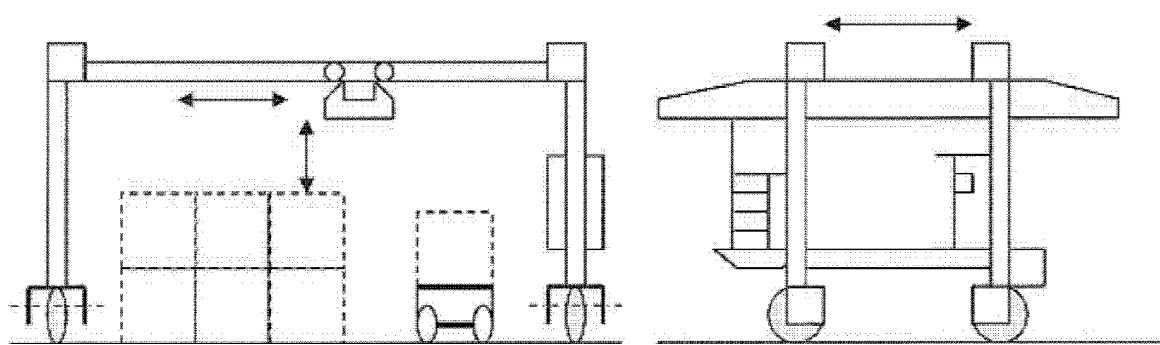
Рисунок 5 - Мостовой портальный контейнерный кран на пневмоходу
