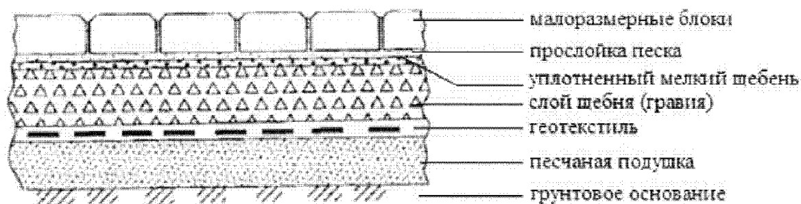
Рисунок 6 - Блочные покрытия
