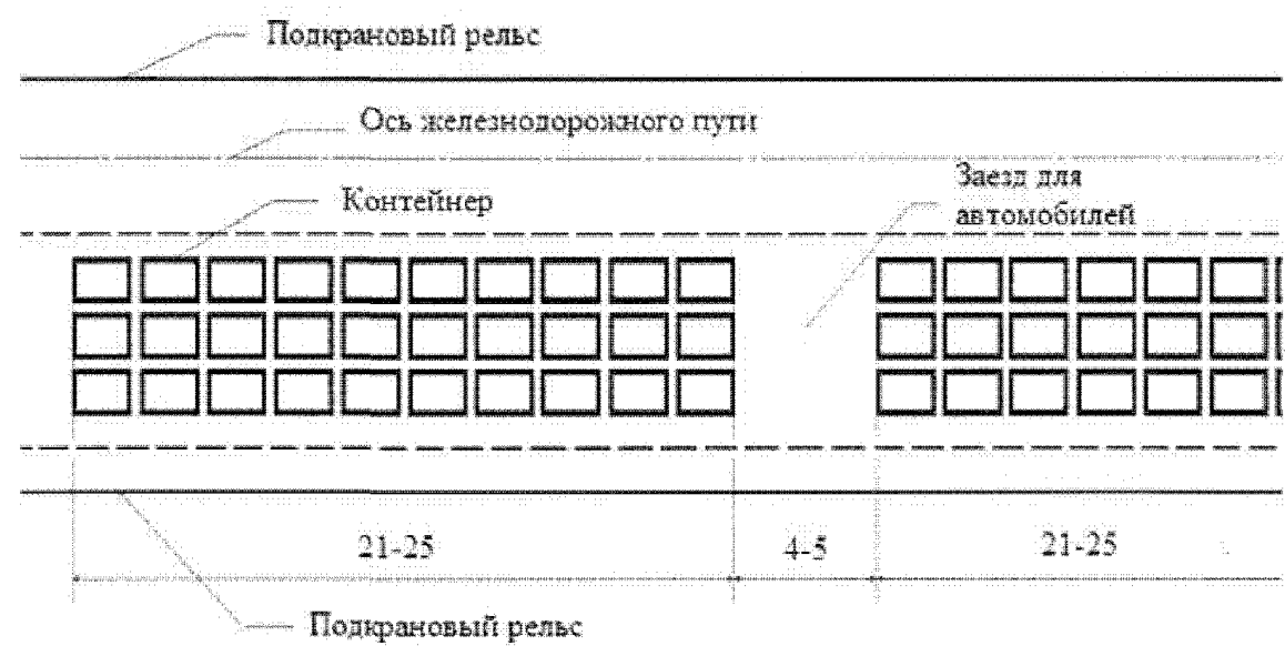
Рисунок 4 - Схема поперечного заезда автомобилей
