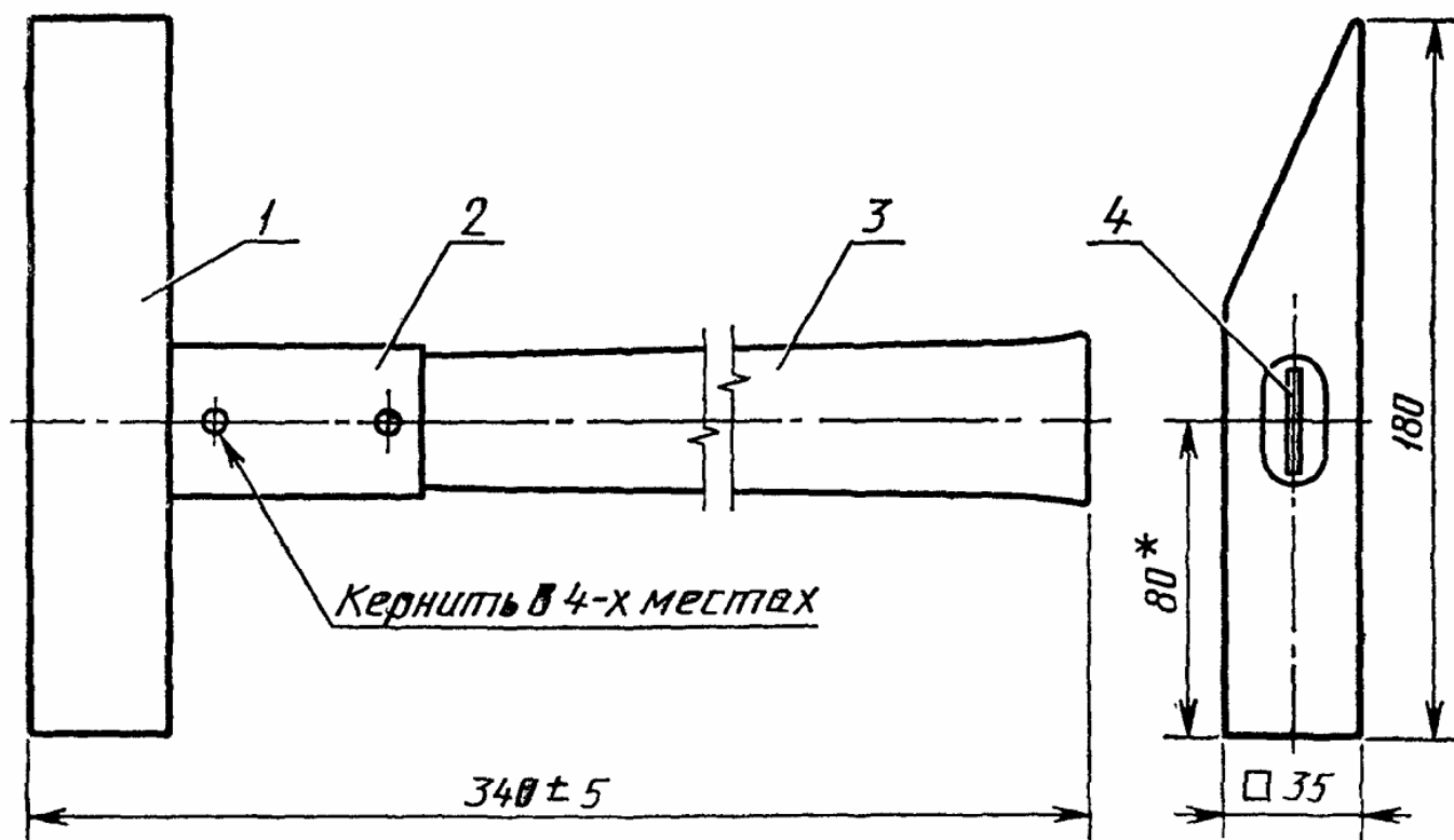
Типоразмер МКР-3
