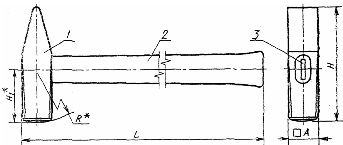
Молотки столярные типа МСТ
