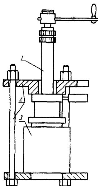
1 - фильтратометр, 2 - крепежное устройство, 3 - бетонный образец
