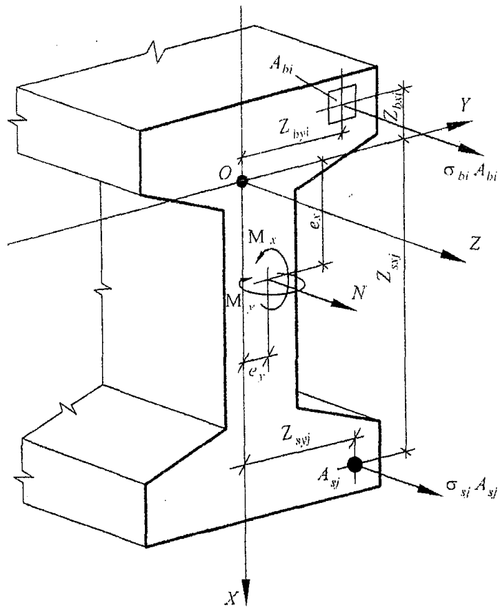
Рисунок 8.5. Расчетная схема нормального сечения железобетонного элемента
