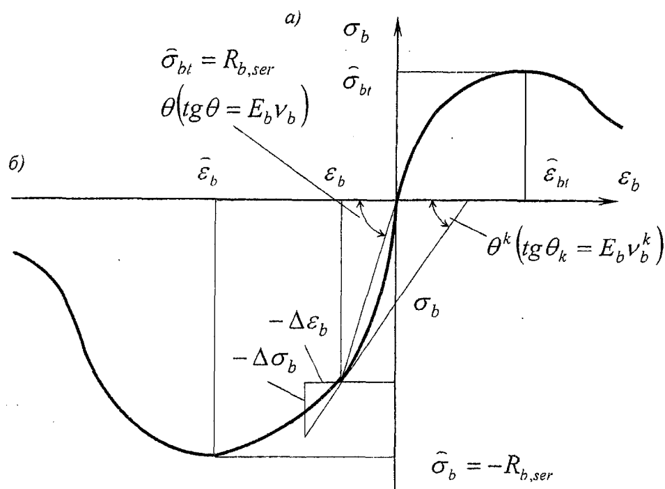
Рисунок Г.1. Криволинейные диаграммы деформирования бетона
