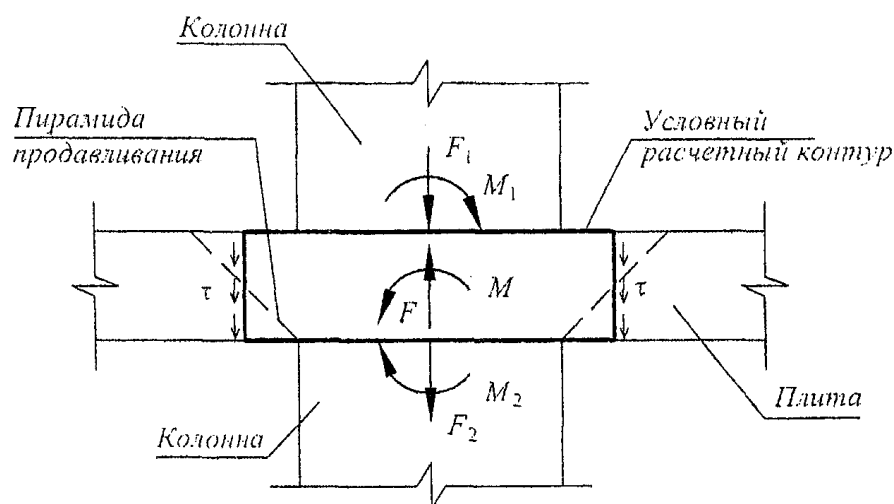
Рисунок 8.10. Условная модель для расчета на продавливание
