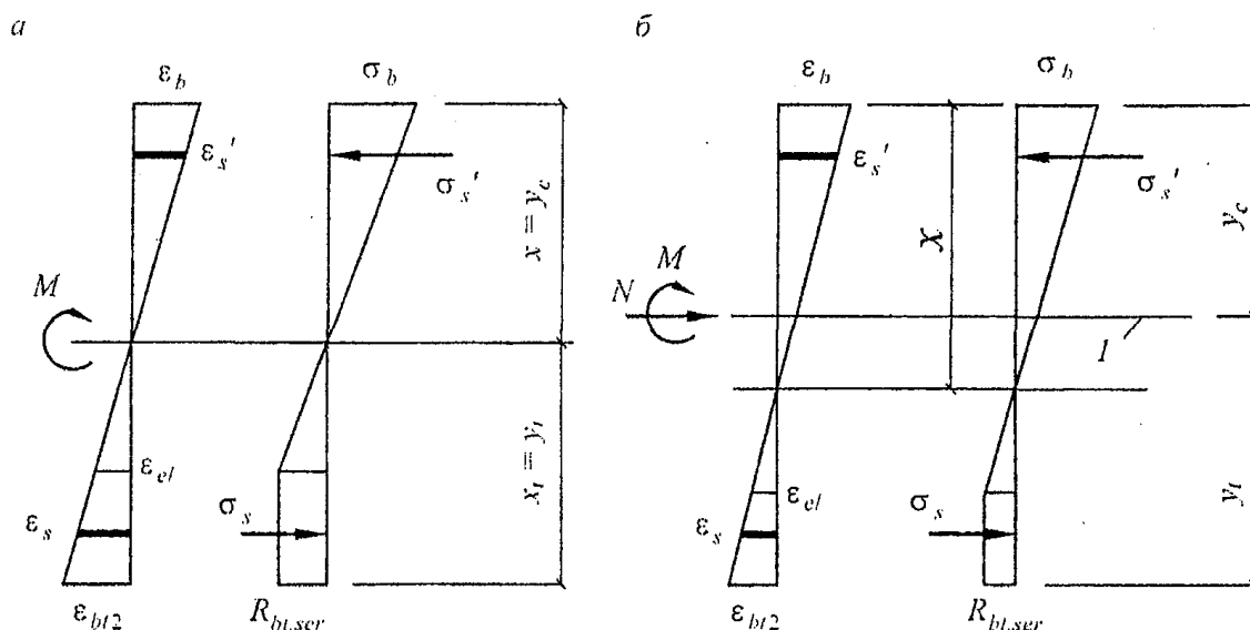
Рисунок 8.17. Схема напряженно-деформированного состояния сечения элемента при проверке образования трещин при действии изгибающего момента (а), изгибающего момента и продольной силы (б)
