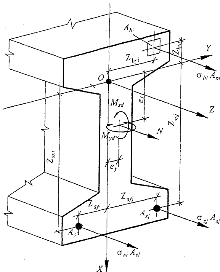
Рисунок 9.2. Расчетная схема нормального сечения
