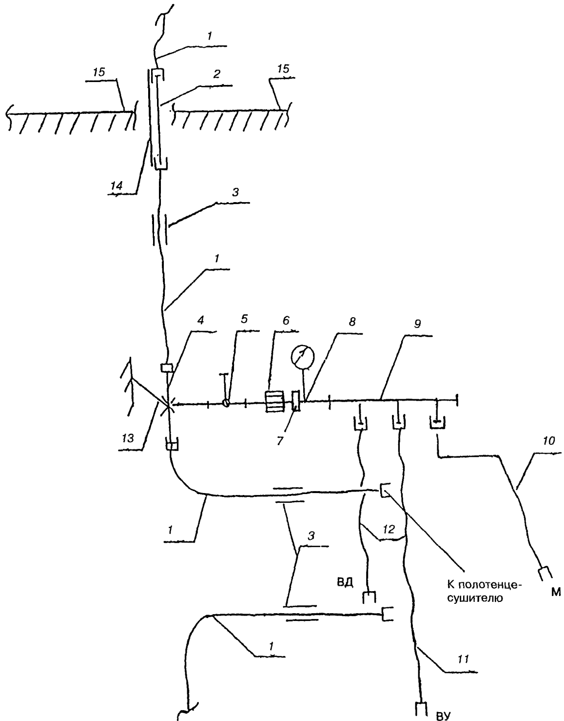
Рисунок 2. Схема этажестояка из МПТ холодного водопровода с распределительным коллектором в сборе с подводками из МПТ.
