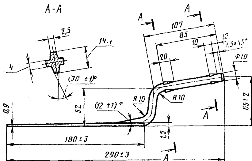
Черт. 8. Полотно с кронштейном цельнокованные кельмы типа КО Исполнение 2
