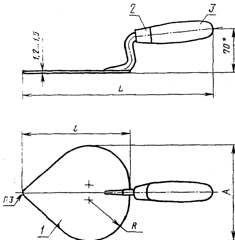
Черт. 4. Кельма типа КШ
