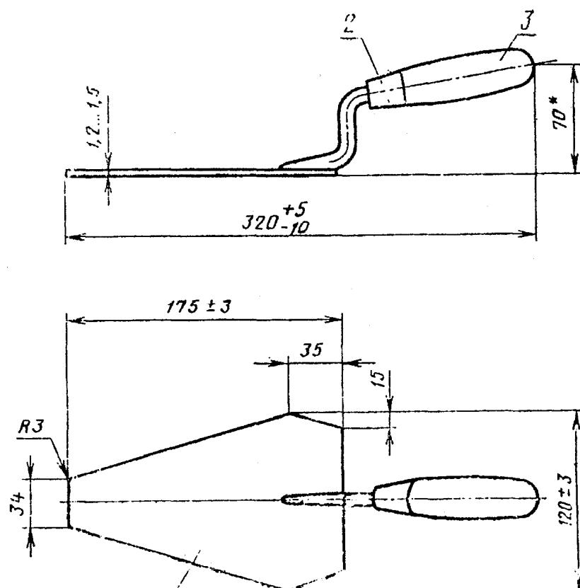
Черт. 6. Лопатка типа ЛП
