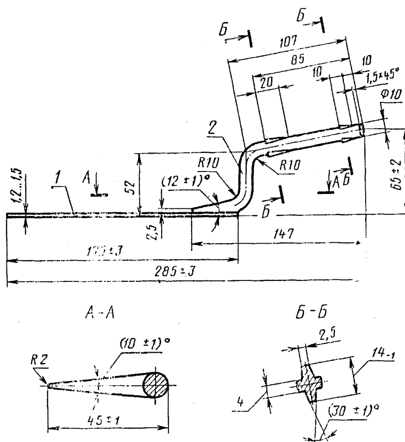
Черт. 9. Полотно с кронштейном кельмы типа ЛП
