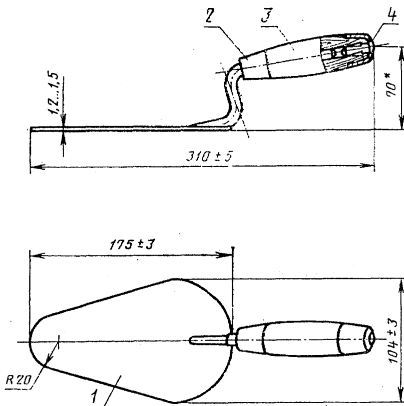
Черт. 3. Кельма типа КП
