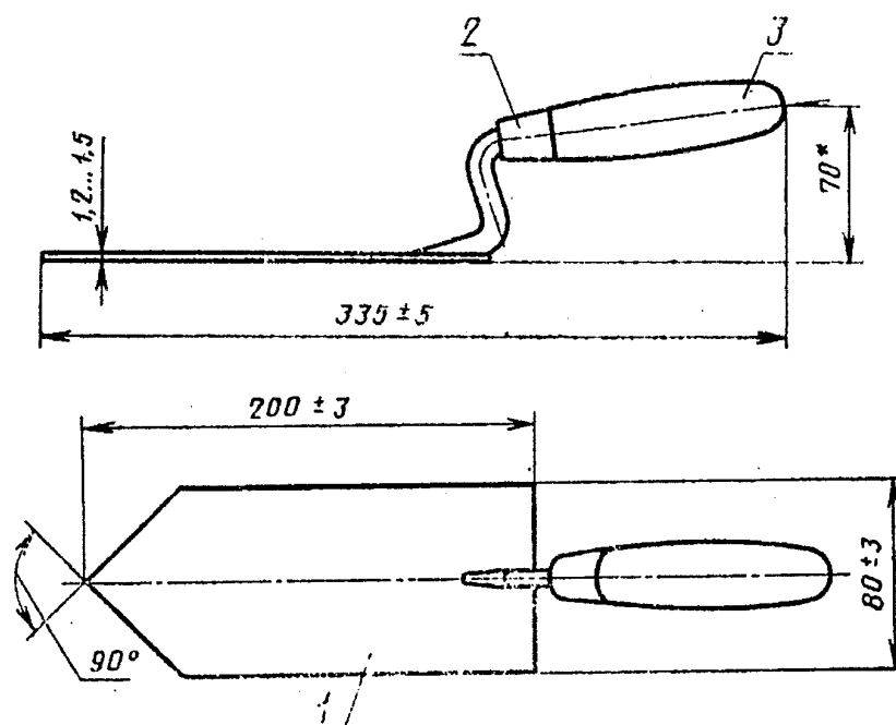
Черт. 7. Лопатка типа ЛК
