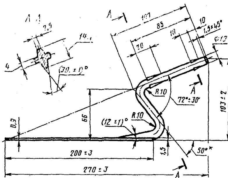
Черт. 2. Полотно с кронштейном цельнокованные кельмы типа КБ Исполнение 2
