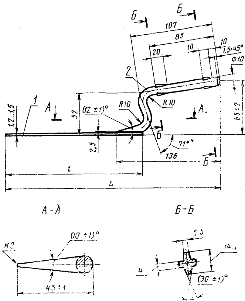
Черт. 6. Полотно с кронштейном кельмы типа КШ
