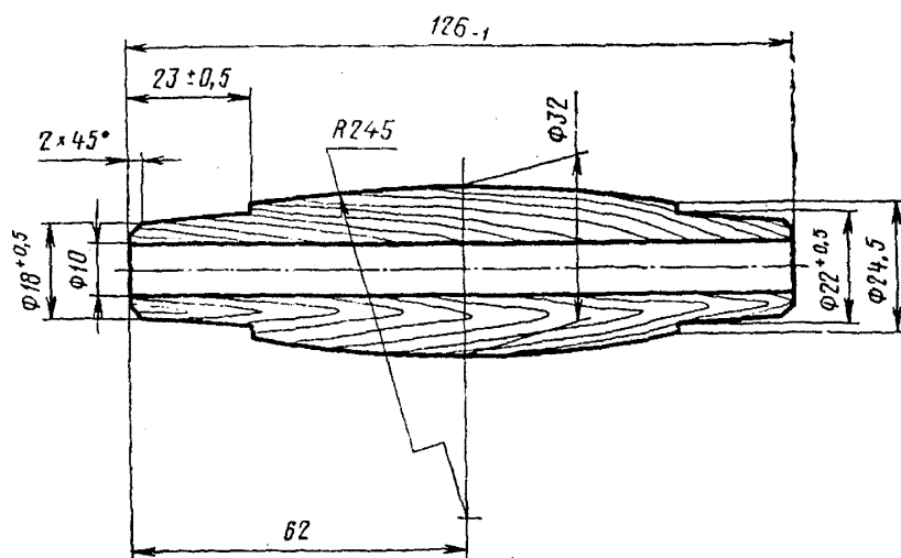
Черт. 12. Ручка для кельм типов КБ и КП
