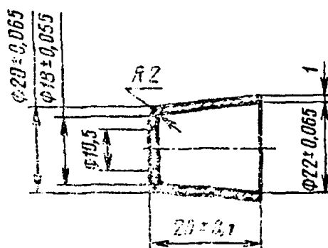
Черт. 15. Колпачок для кельм и лопаток
