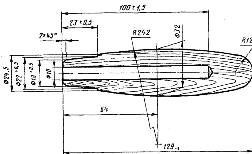
Черт. 14. Ручка для кельм типов КШ, КО и лопаток типов ЛК и ЛП
