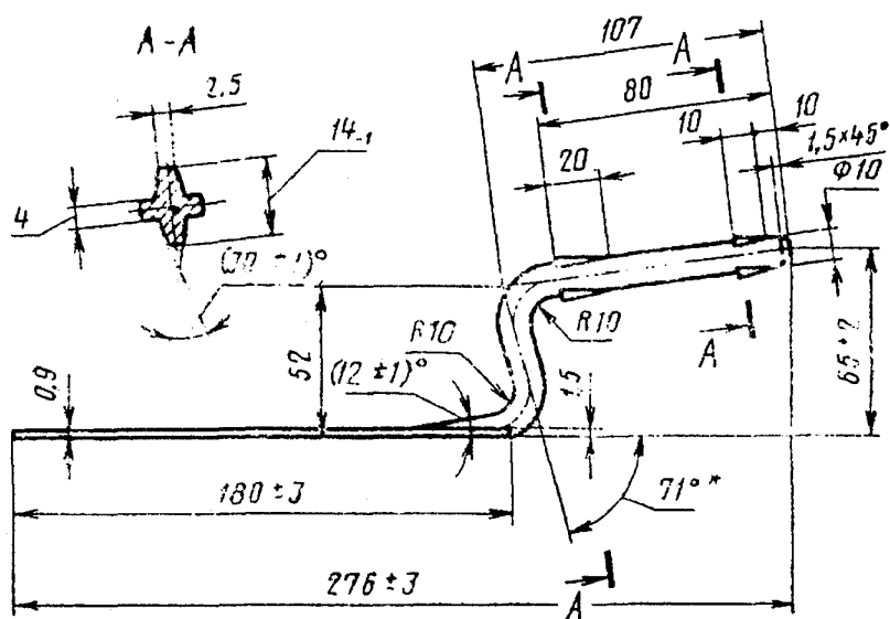
Черт. 5. Полотно с кронштейном цельнокованные кельмы типа КП
