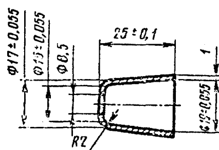
Черт. 17. Колпачок для отрезки
