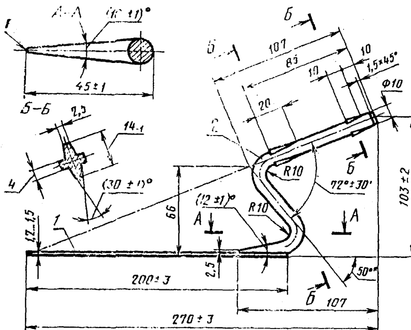
Черт. 1. Полотно с кронштейном кельмы типа КБ Исполнение 1
