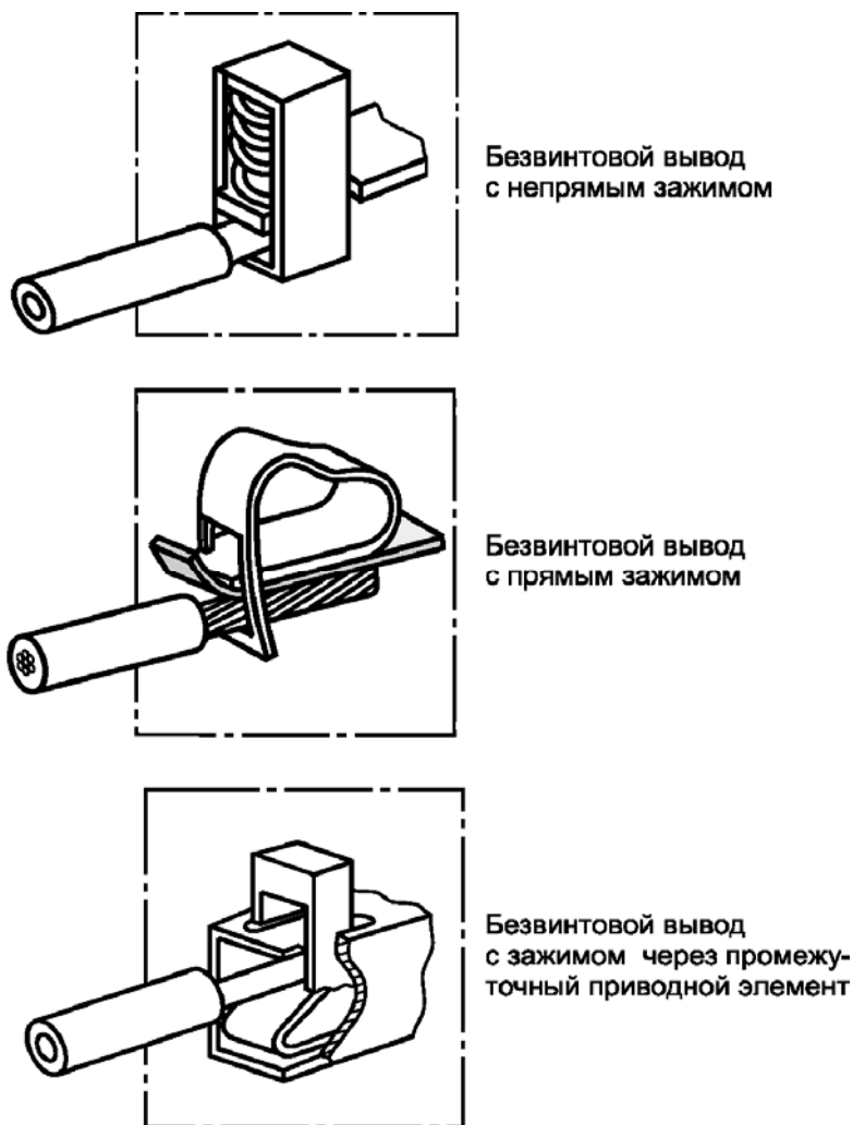
Рисунок J.2. Примеры безвинтовых выводов
