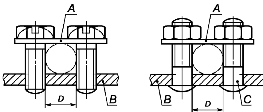
Рисунок F.2. Пример винтовых и штыревых выводов
