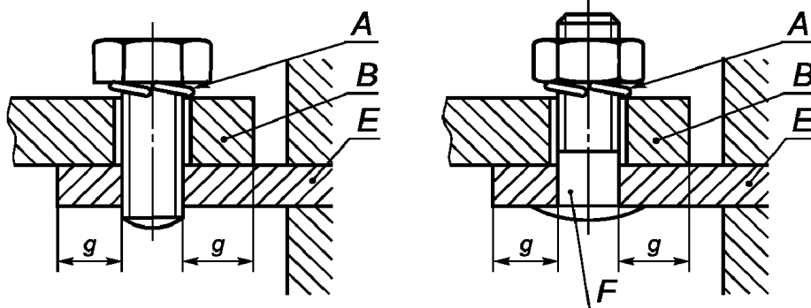
А - запорное устройство; В - кабельный наконечник или шина; Е - неподвижная часть; F - штырь
