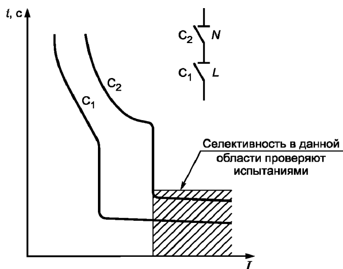
Рисунок D.1. Координация по сверхтокам между автоматическим выключателем и предохранителем или резервной защитой, осуществляемой предохранителем. Рабочие характеристики
