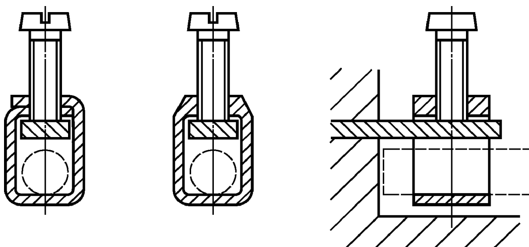
Выводы с хомутиком
