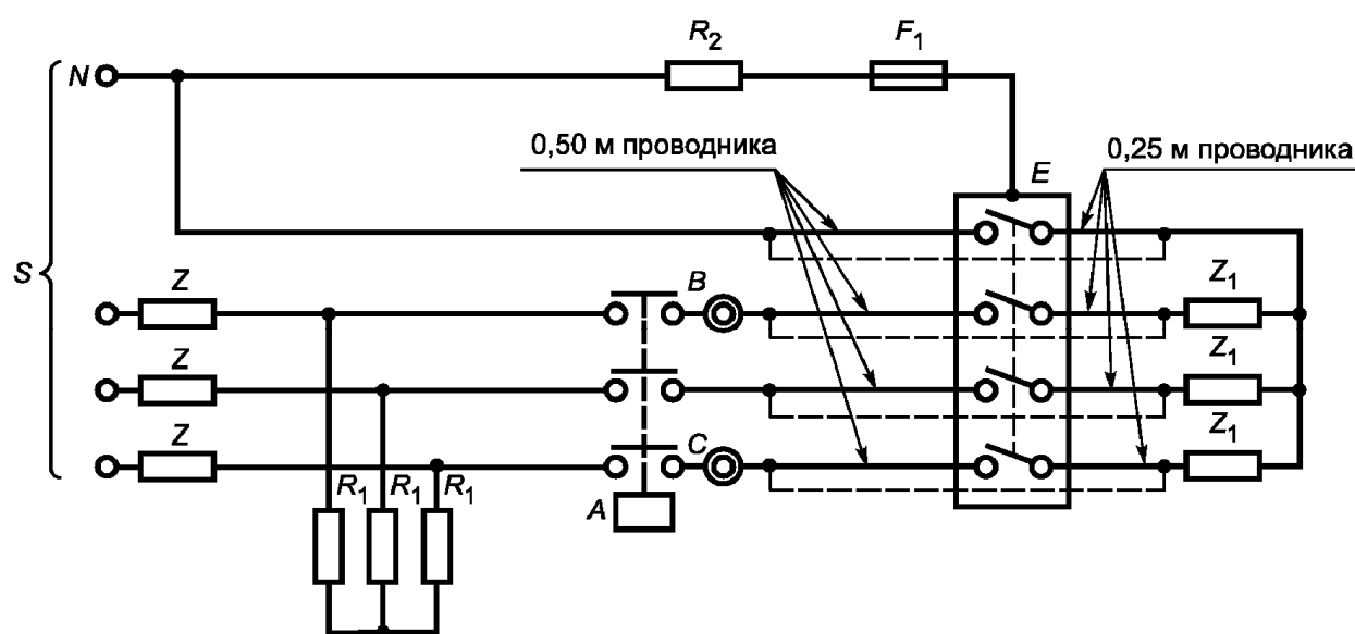
Рисунок 6. Четырехполюсный автоматический выключатель
