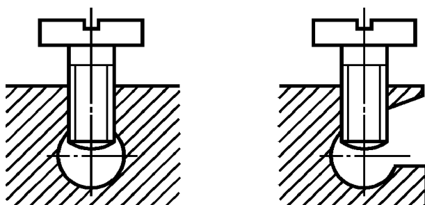
Выводы без прижимных пластин
