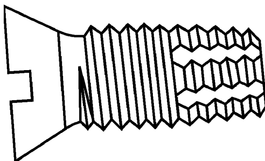
Рисунок 2. Самонарезающий режущий винт (3.3.23)
