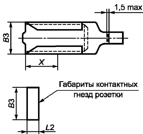
Рисунок К.5. Размеры отверстий для фиксации
