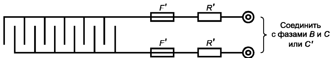
Рисунок Н.3. Цепь решетки
