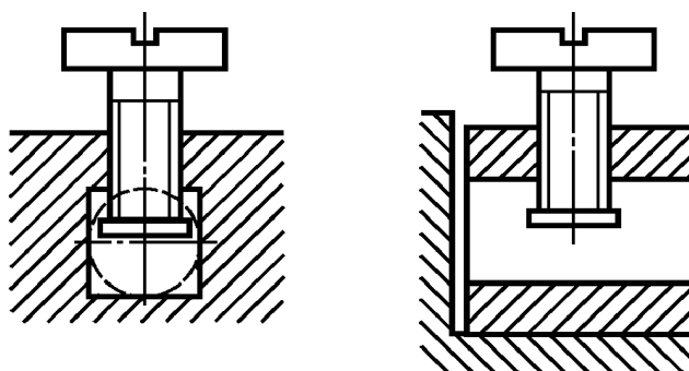
Выводы с прижимными пластинами
