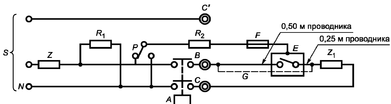
Рисунок 3. Однополюсный автоматический выключатель
