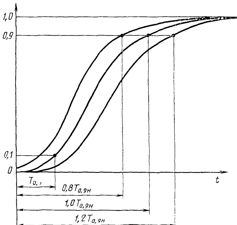
ГРАФИК ПЕРЕХОДНОГО ПРОЦЕССА
