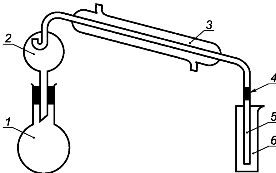
1 - круглодонная колба; 2 - каплеуловитель; 3 - стеклянный лабораторный холодильник; 4 - резиновая трубка; 5 - стеклянная отводная трубка; 6 - цилиндр для приема дистиллята
