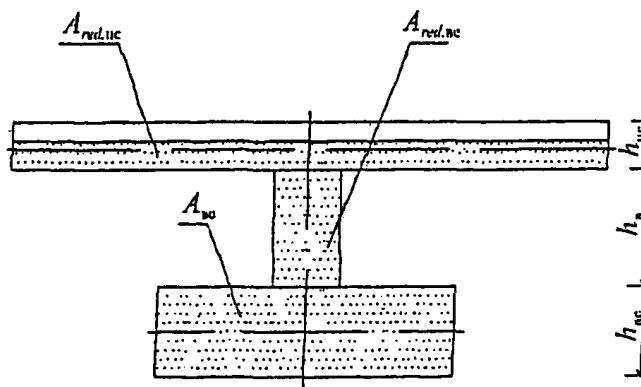
Рисунок 10. Приведенное сечение рассчитываемого фрагмента стены
