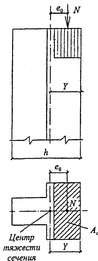
Рисунок 5. Внецентренное сжатие
