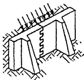
Рисунок 3. Растяжение кладки при изгибе по перевязанному сечению
