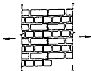
Рисунок 2. Растяжение кладки по перевязанному сечению
