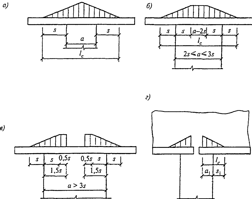
а - на средних опорах неразрезных балок при a \leq 2s ; б - то же, при 3s \geq a > 2s ; в - то же, при a > 3s ; г - на крайних опорах неразрезных балок и на опорах
