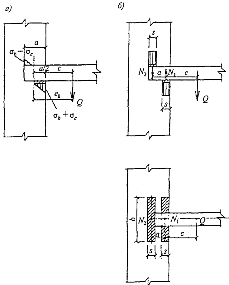
Рисунок 14. Расчетные схемы заделки консольных балок
