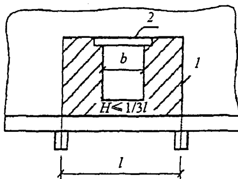
1 - нагрузка на рандбалку; 2 - железобетонная перемычка
