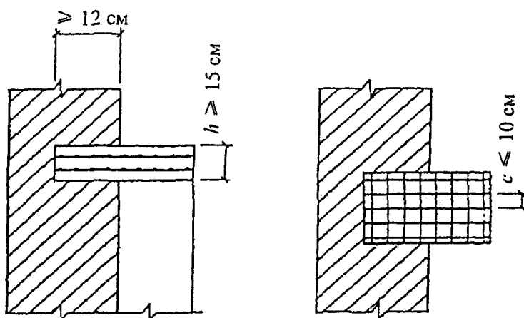
Рисунок 13. Железобетонные распределительные плиты
