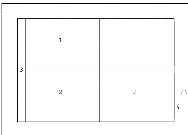
Рисунок А.4. Схема раскроя точечных проб тканей (испытание по ГОСТ 3813 и ГОСТ 17922 ) и трикотажных полотен и изделий
