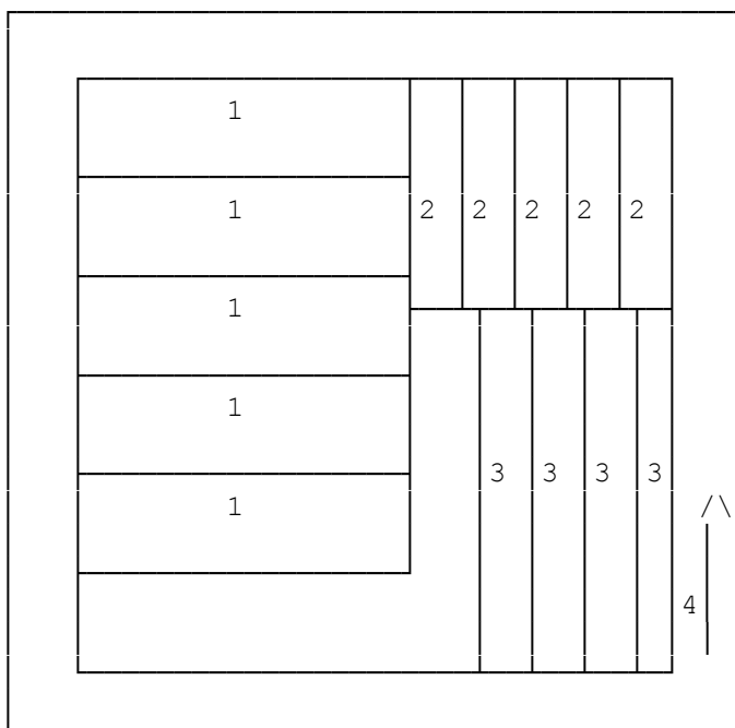
Рисунок А.8. Схема раскроя точечной пробы нетканого материала (1-я часть)
