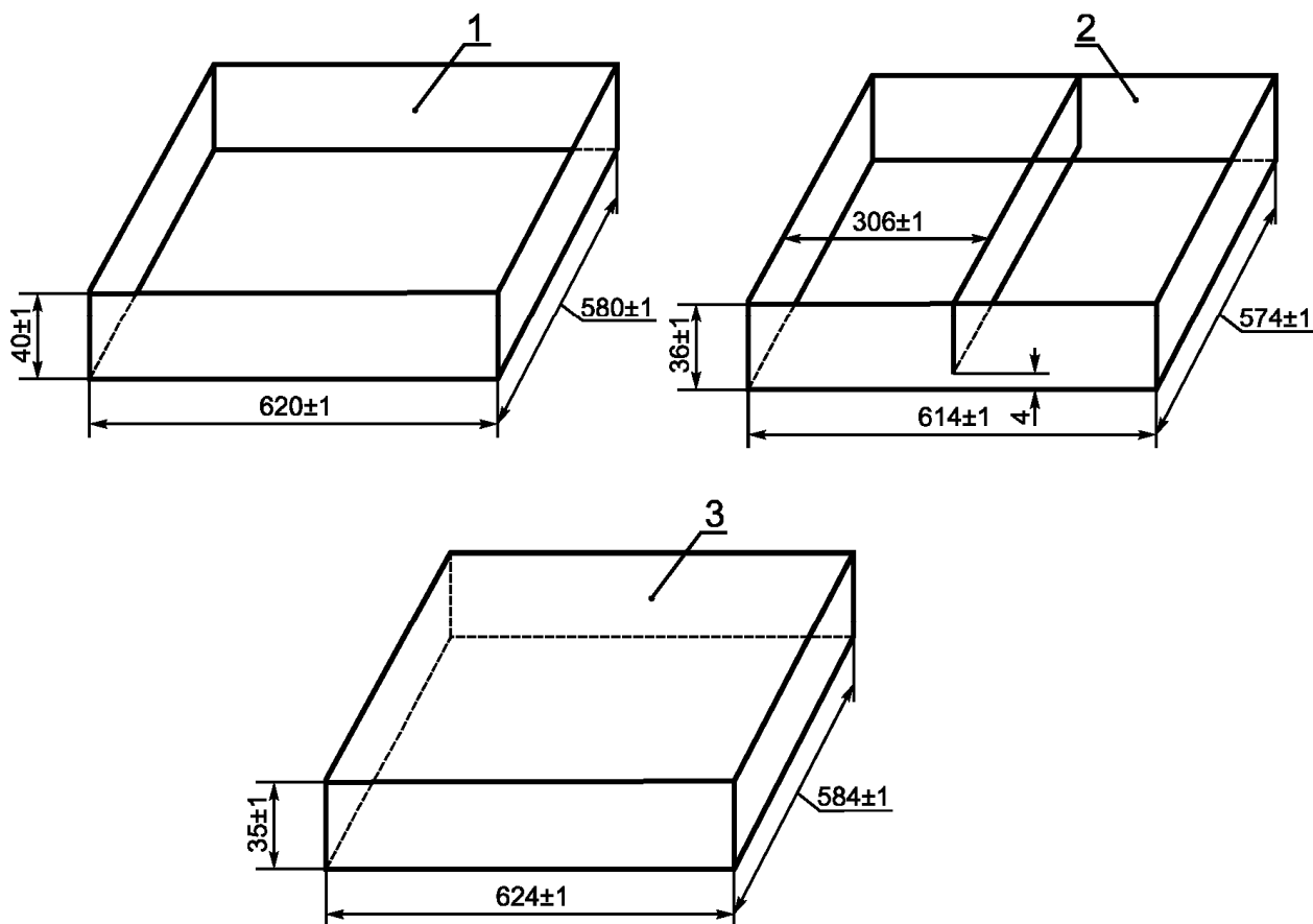
1 - кювета; 2 - рамка; 3 - крышка
