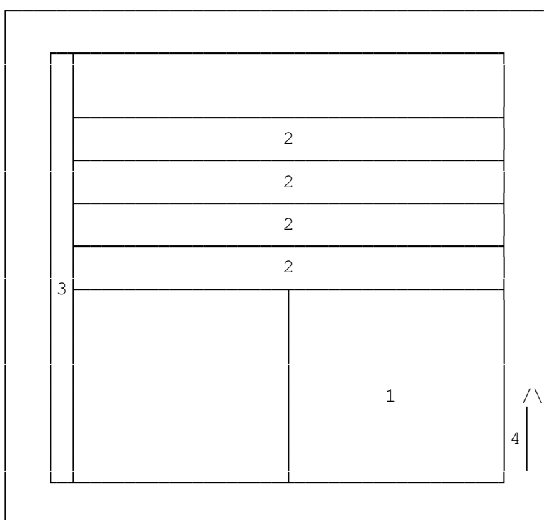
Рисунок А.6. Схема раскроя точечной пробы (2-я часть) технической ткани (испытание по ГОСТ 29104.4 и ГОСТ 29104.5 )
