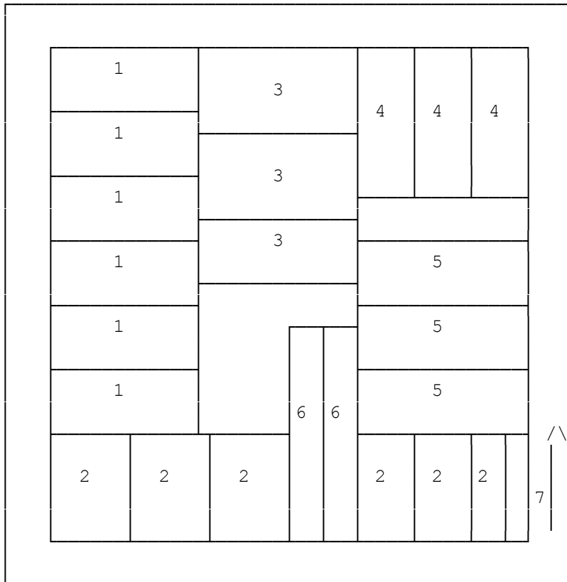
Рисунок А.1. Схема раскроя точечной пробы прорезиненной ткани
