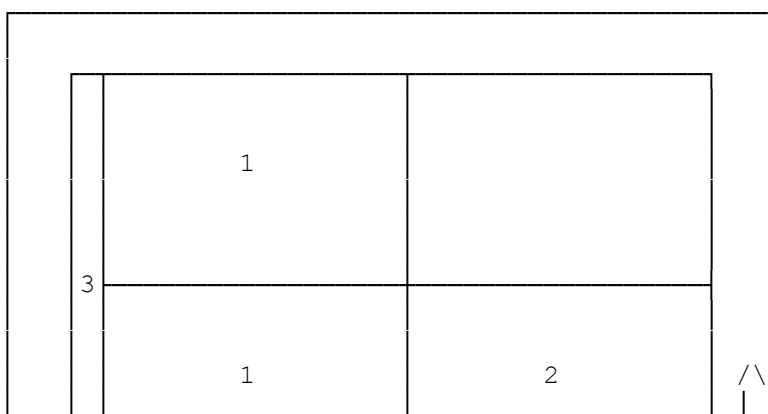
Рисунок А.5. Схема раскроя точечной пробы (1-я часть) технической ткани (испытание по ГОСТ 29104.4 и ГОСТ 29104.5 )
