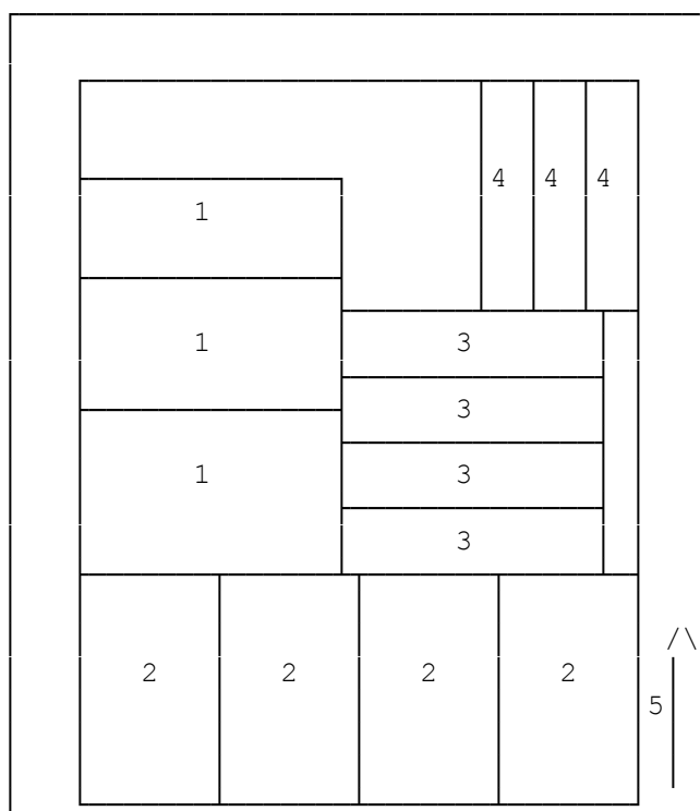
Рисунок А.3. Схема раскроя точечной пробы искусственной кожи
