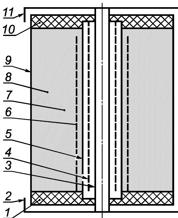
Рисунок А.1. Схематический разрез вертикальной печи сопротивления
