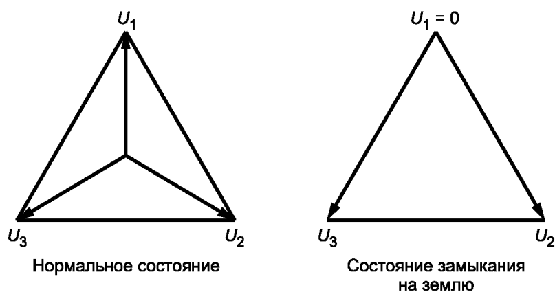
Рисунок С.2. Напряжения на испытуемом счетчике
