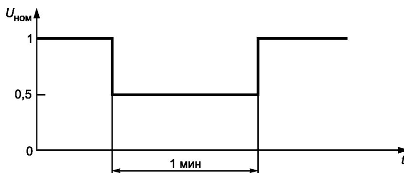
Рисунок В.3. Провалы напряжения \Delta U = 50\%
